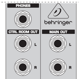
图 2.9: 监听混音 / 主混音接口
