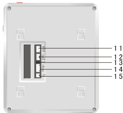
后视图
