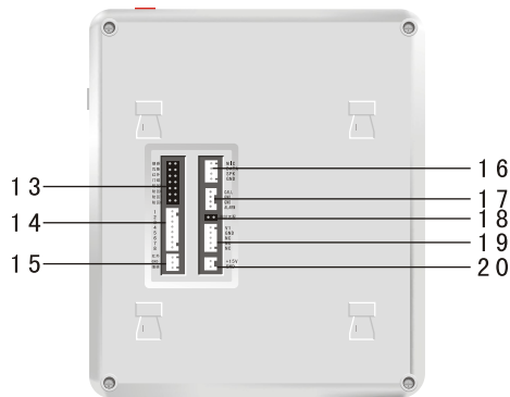
后视图
