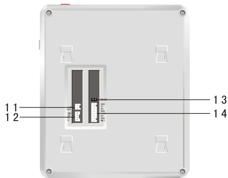
后视图
