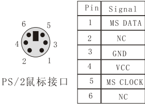
PS/2鼠标接口针脚定义
