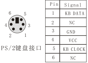
PS/2键盘接口针脚定义
