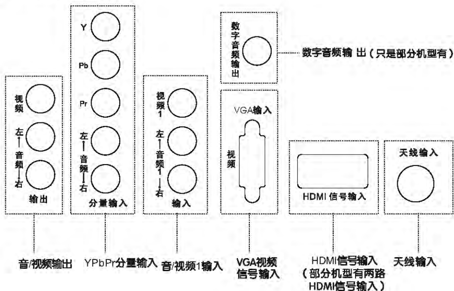
后AV端子示意图
