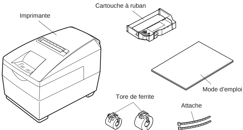
Fig. 2-1 Déballage
