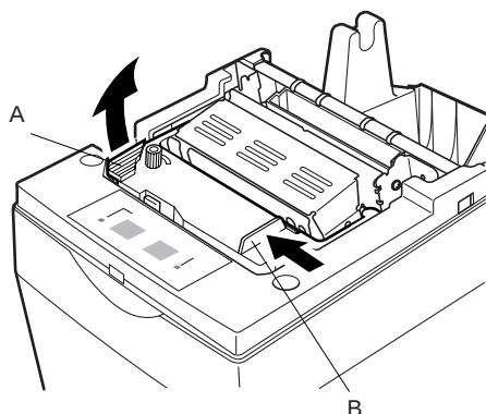
Abb. 6-3 Farbbandkassette ausbauen
