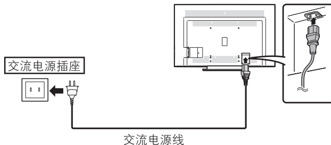
电视机 (后视图)
