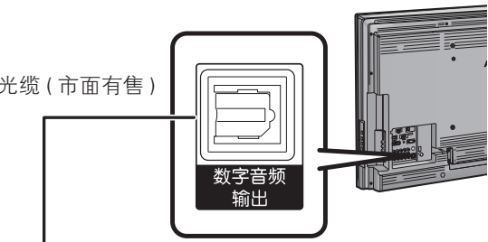
连接到外接音频设备的光学数码输入
