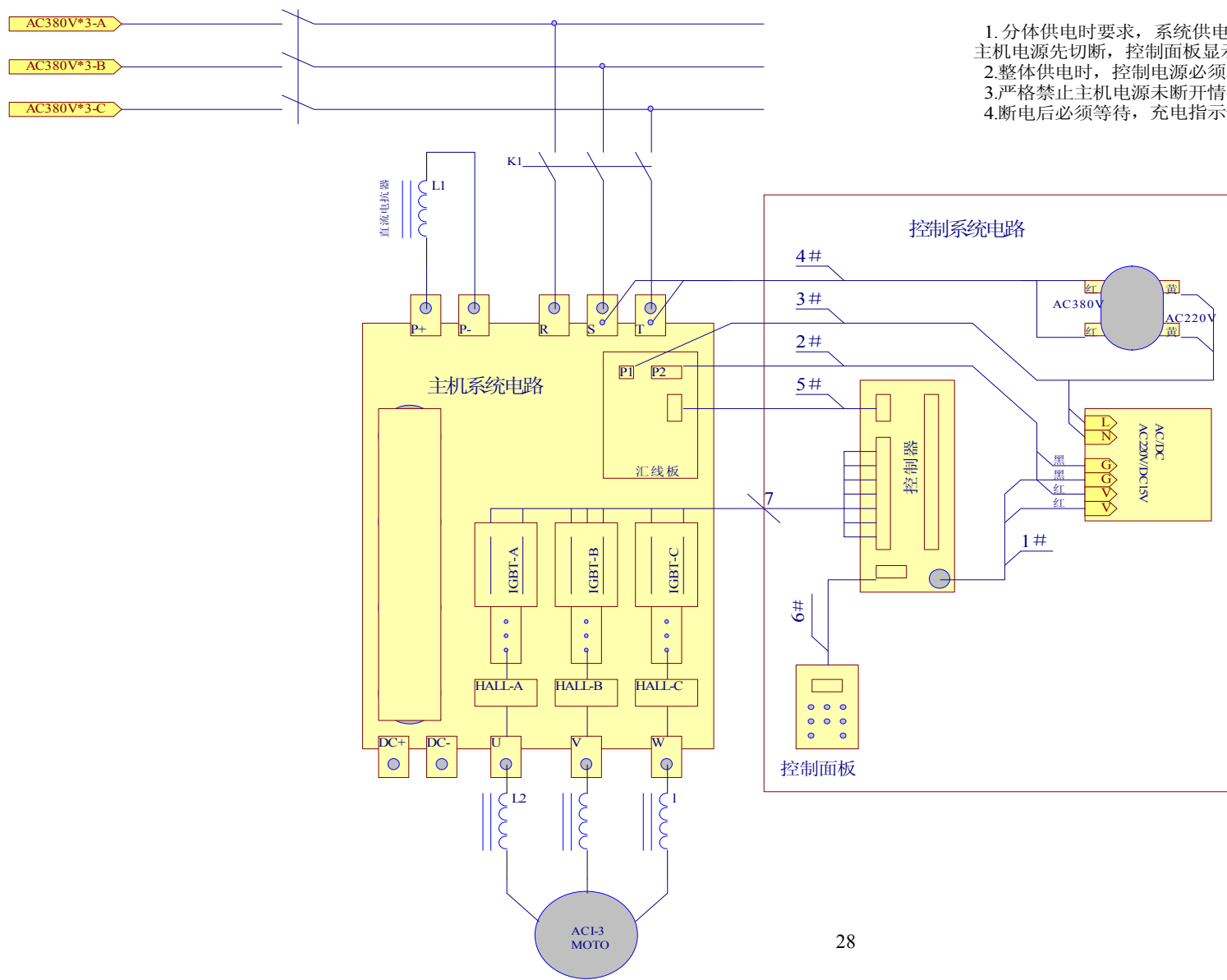
SC800 接外部接线图—整体供电
