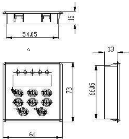
面板尺寸图
