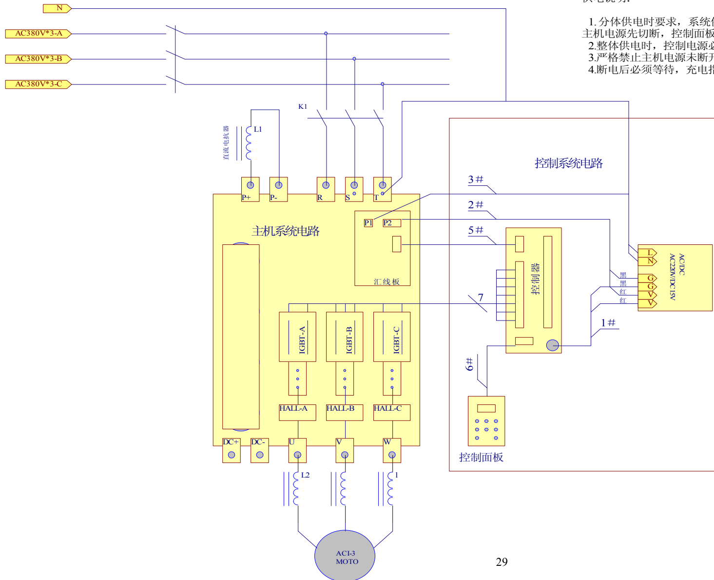
SC800 接外部接线图——不带变压器的整体供电电路
