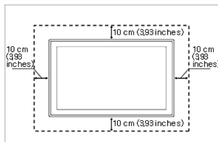
使用壁挂支架安装产品时
