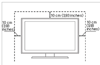
使用底座支架安装产品时
