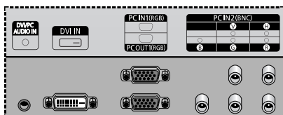
PDP 显示器的背面
