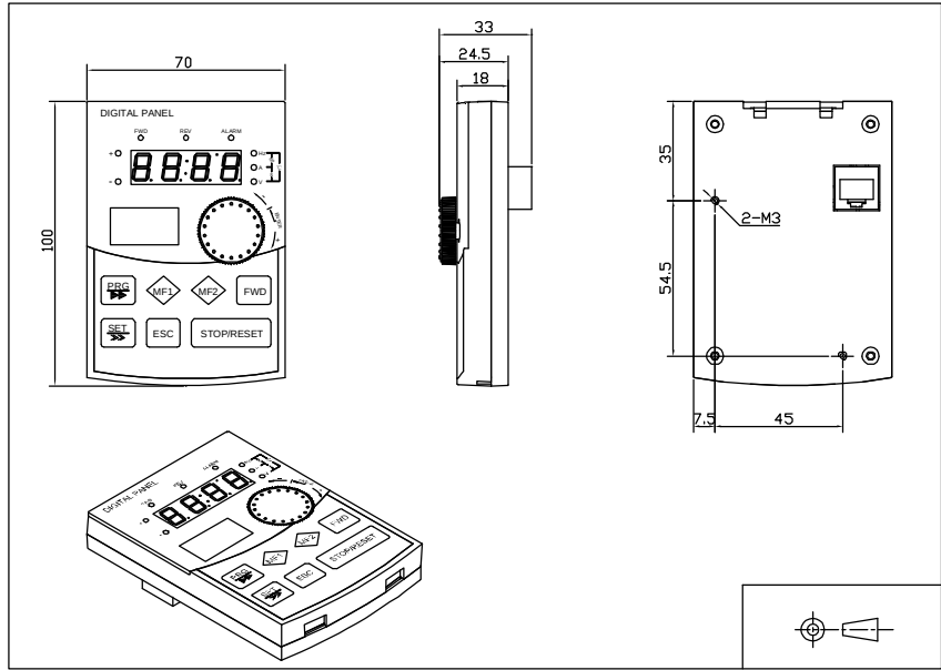
JP6E8000 尺寸图:
