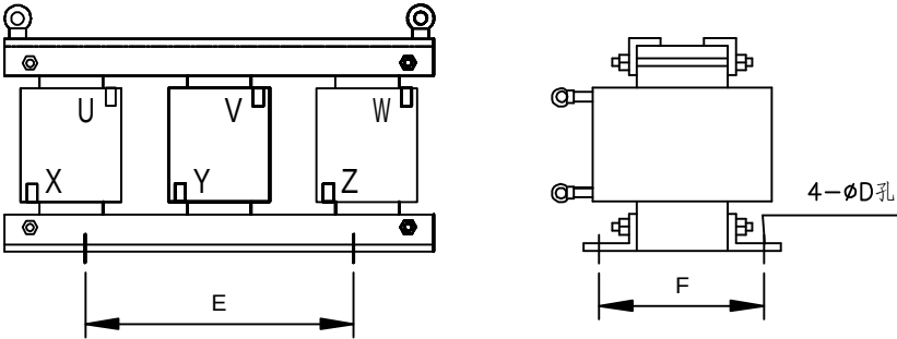
外形尺寸：
