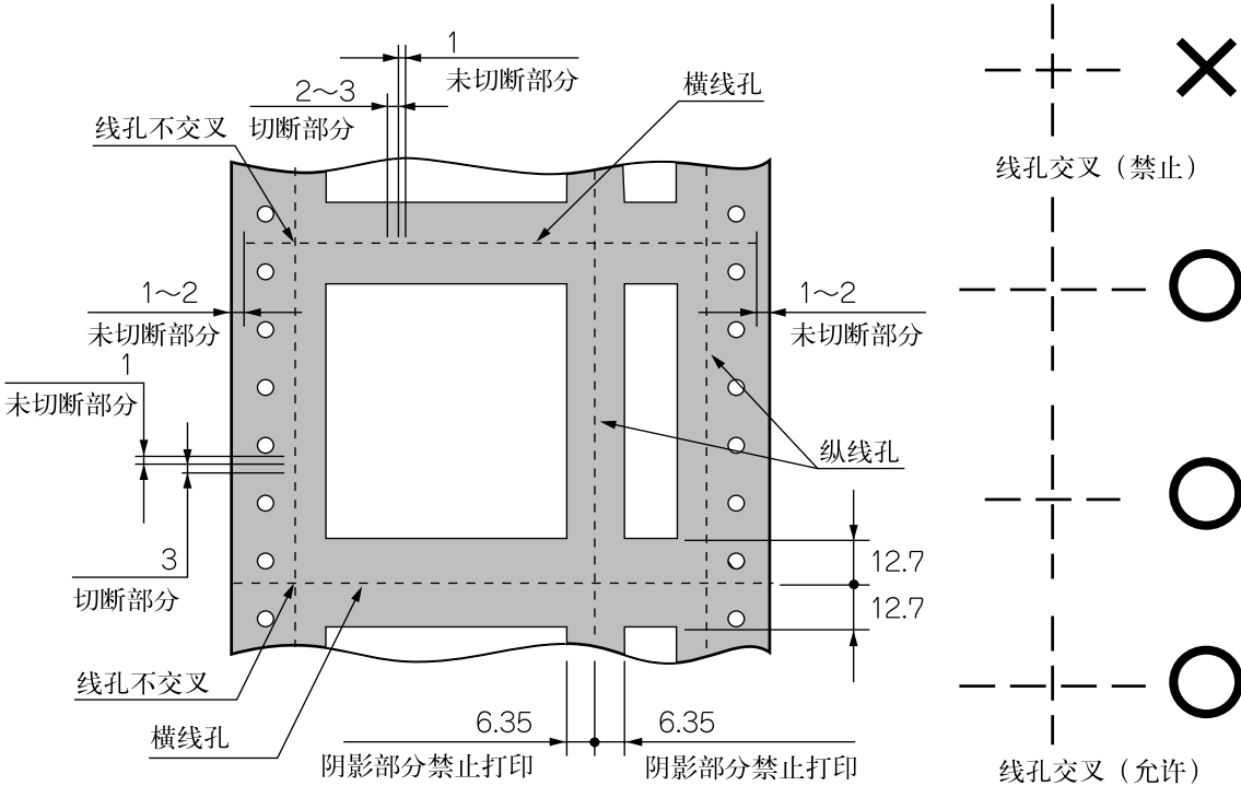
单位：mm
