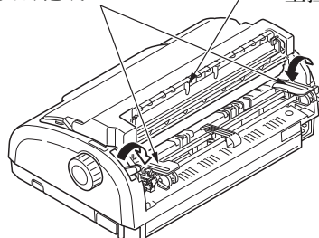
突脚拖纸器盖 上拉导纸器
