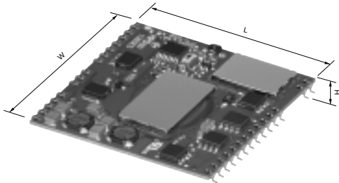
MPD6D12*S系列 MPD7D05*S/13*S/12*S系列
