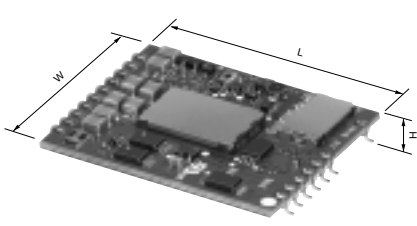
MPD6D10*S/11*S/20*S系列 MPD7D06*S系列
