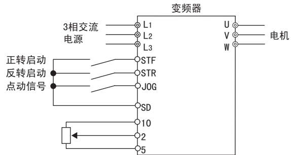
外部点动运行的接线图示例
