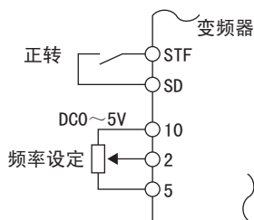
使用端子2 (DC0~5V) 的接线图
