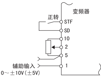
加算补偿接线图
