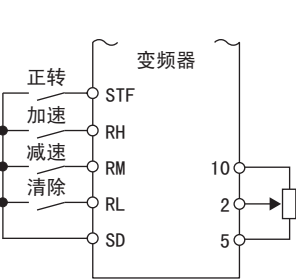
遥控设定的接线图示例
