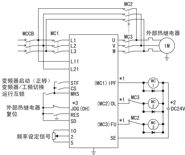
工频切换顺序接线图
