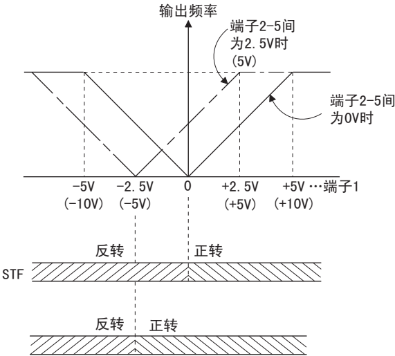
(b) Pr. 73的设定值为10~15时
