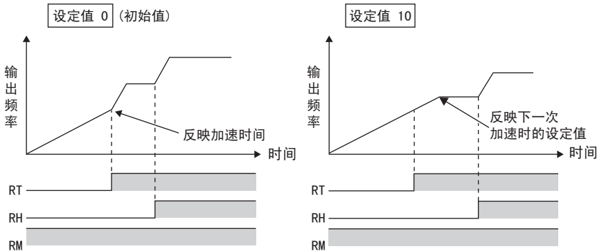
第二加减速时间示例
