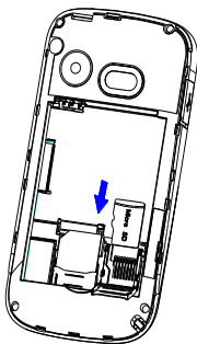
SD 卡的安装朝向示意图
