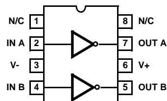
ICL7667 (PDIP, SOIC) TOP VIEW
