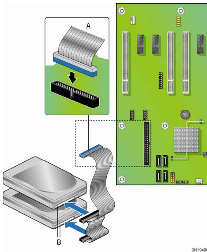
图 18. 连接 IDE 电缆
