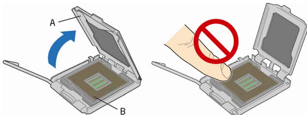
图 7. 抬起压板
