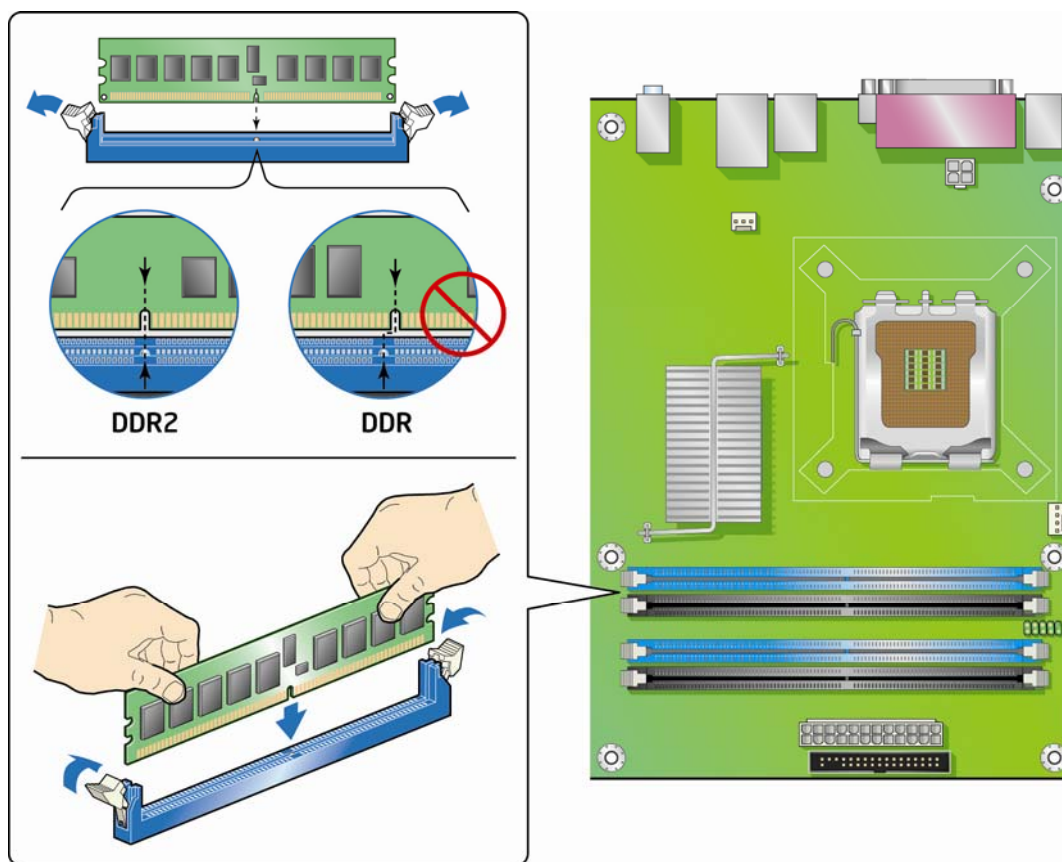
图 17. 安装 DIMM
