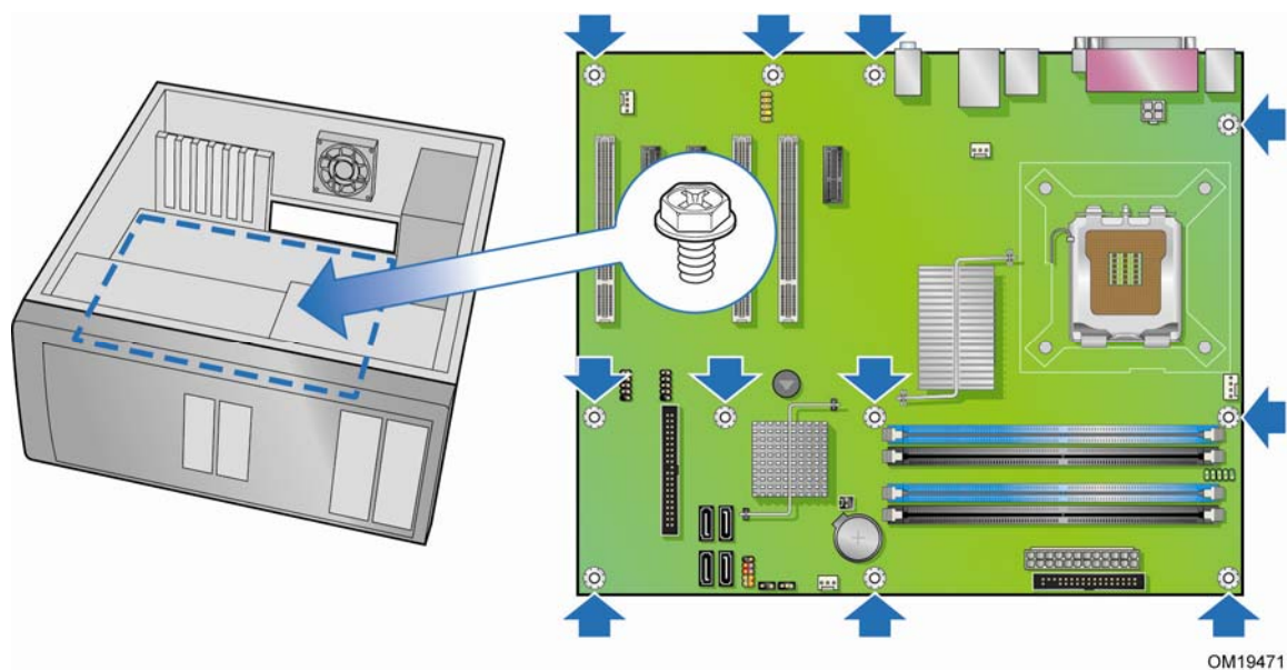
图 5. 台式机主板 DQ963FX 安装螺丝孔位置
