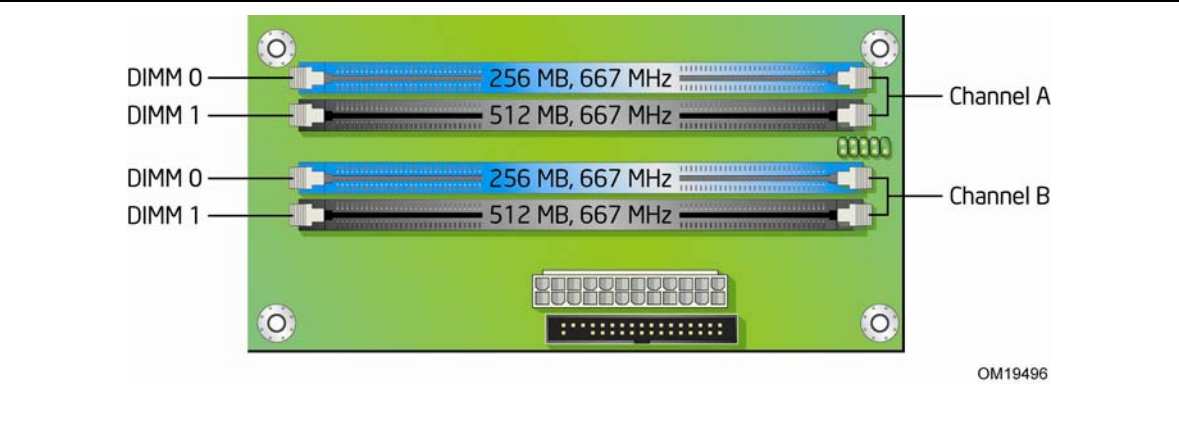
图 14. 双通道内存配置示例 2
