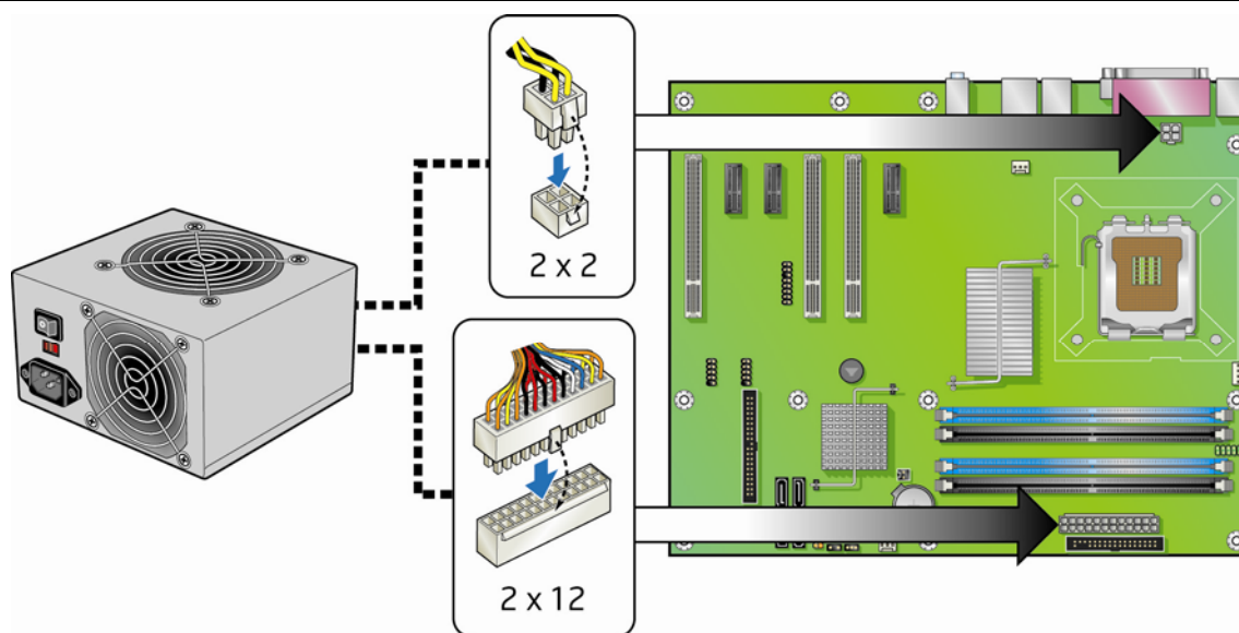
图 23. 连接电源系统电缆
