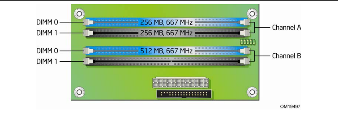
图 15. 双通道内存配置示例 3
