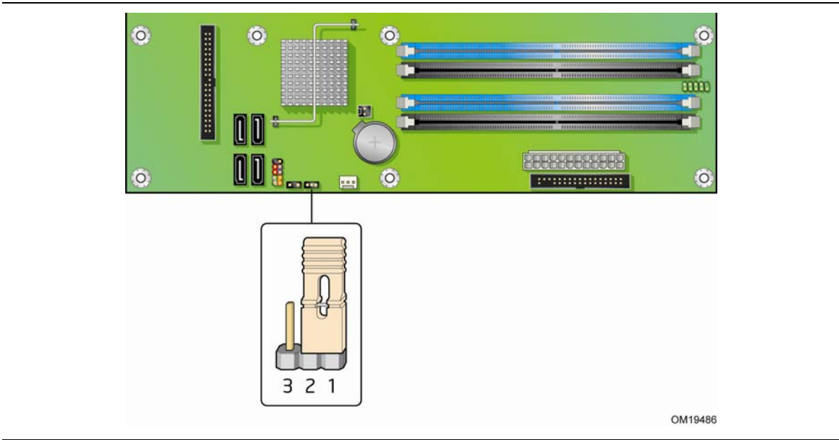
图 25. BIOS 配置跳线块位置
