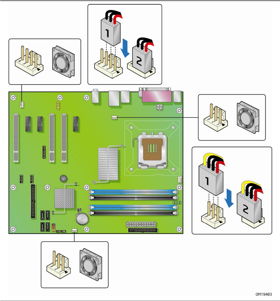
图 22. 机箱风扇接头连接器位置
