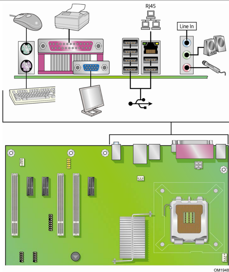
图 26. 背面板连接器
