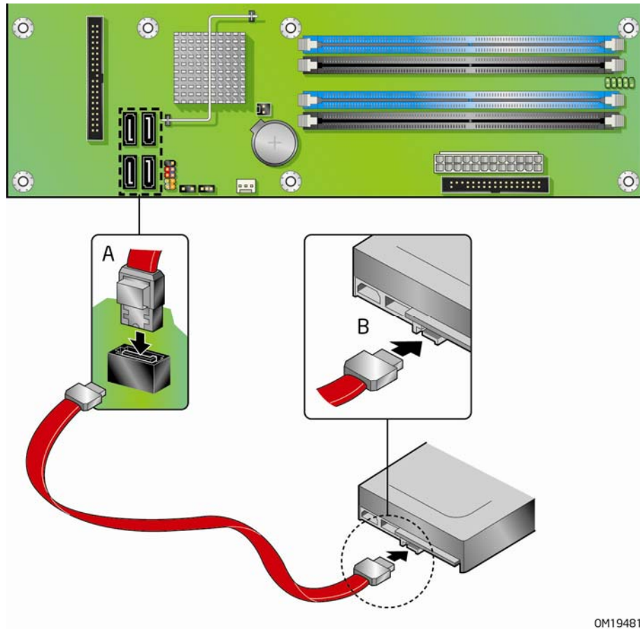
图 19. 连接串行 ATA 电缆
