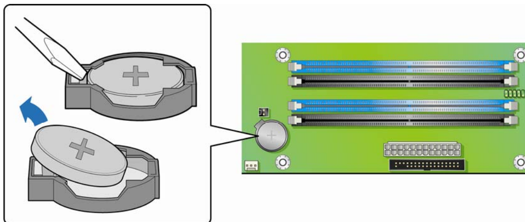
图 27. 拆卸电池
