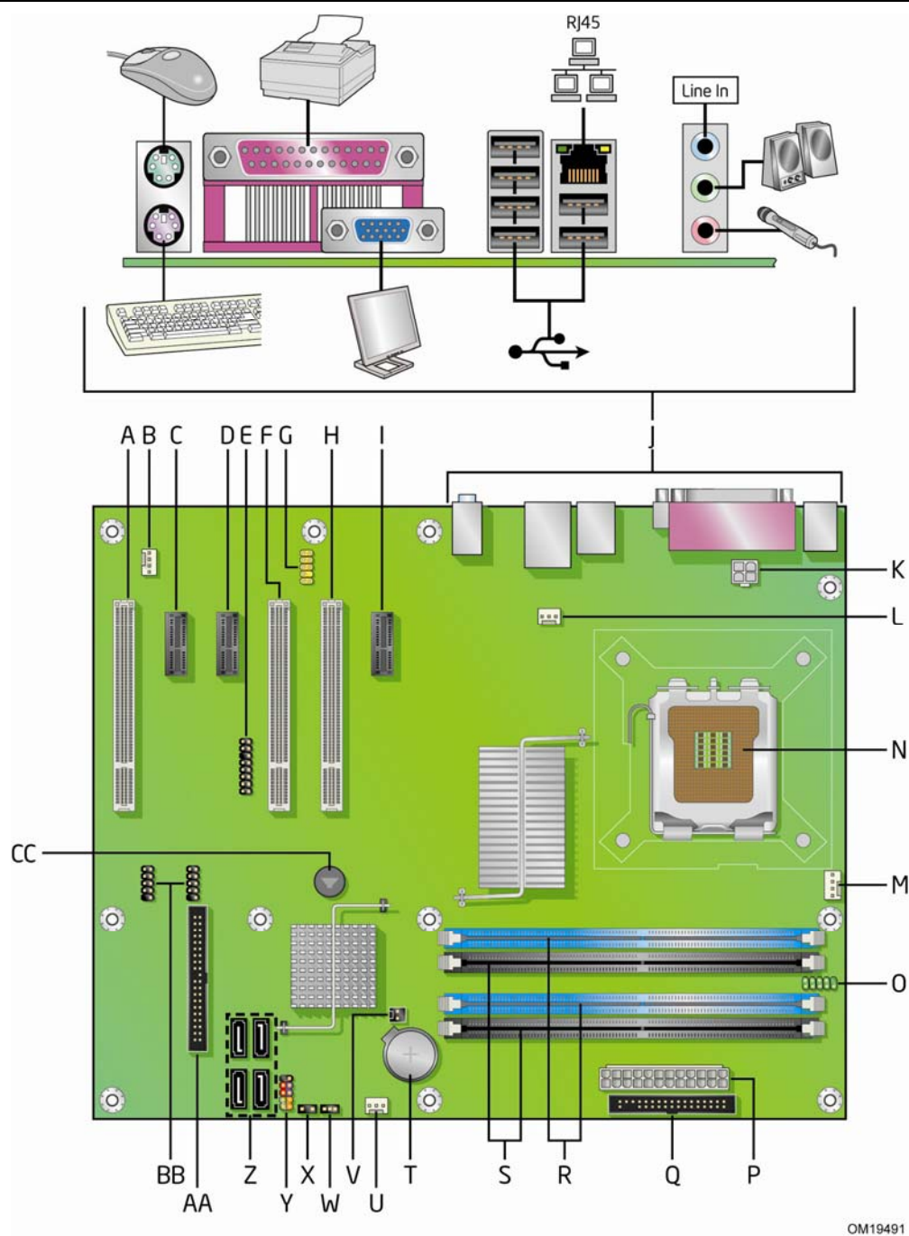
图 1. 台式机主板 DQ963FX 组件
