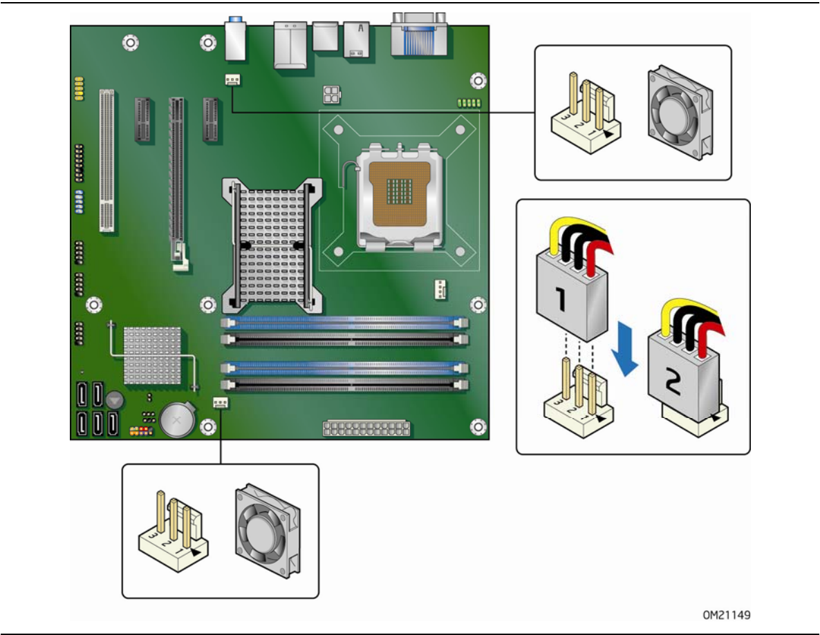
图 24. 机箱风扇接头连接器位置
