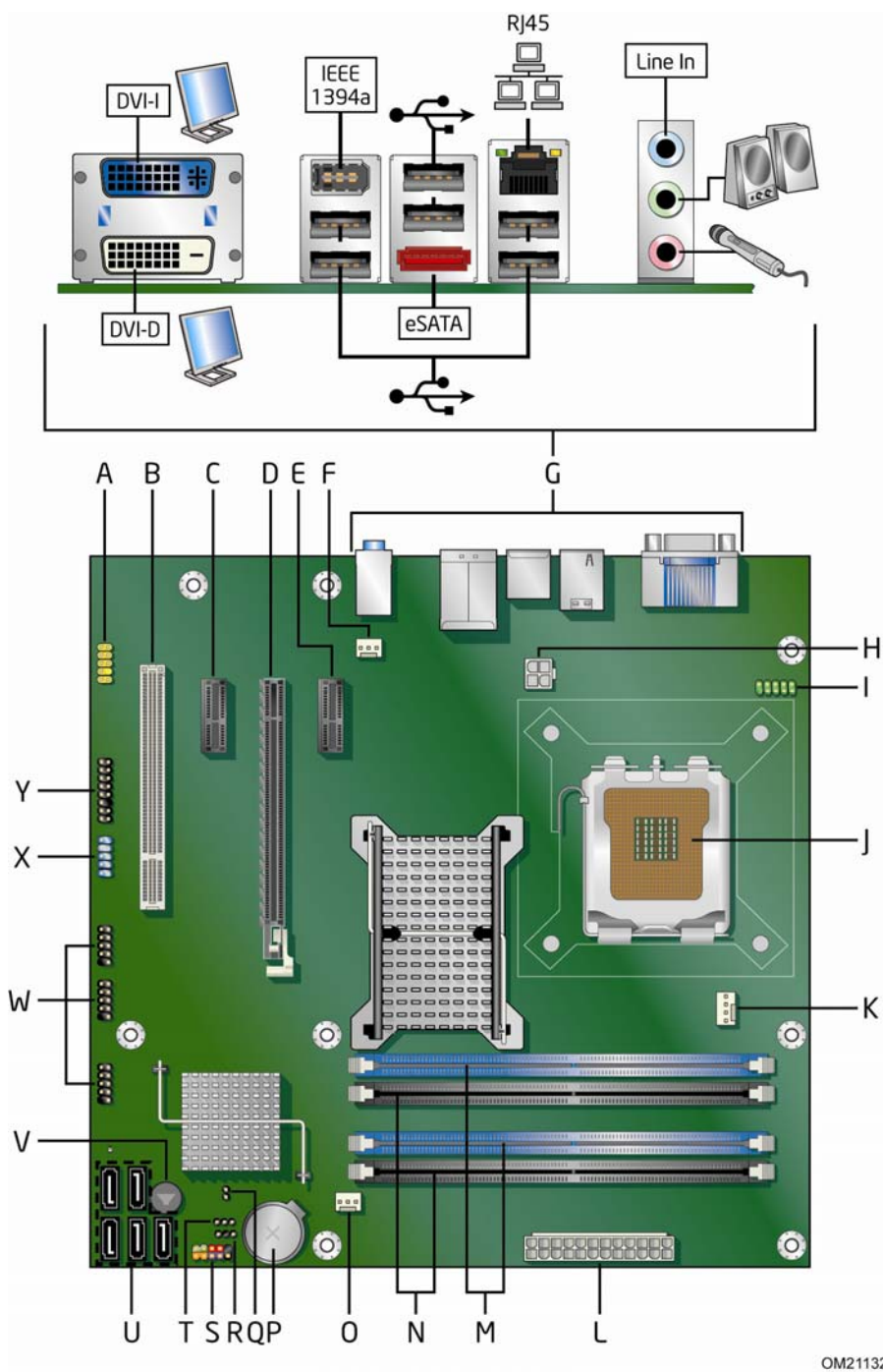
图 1. 英特尔台式机主板 DQ45CB 组件
