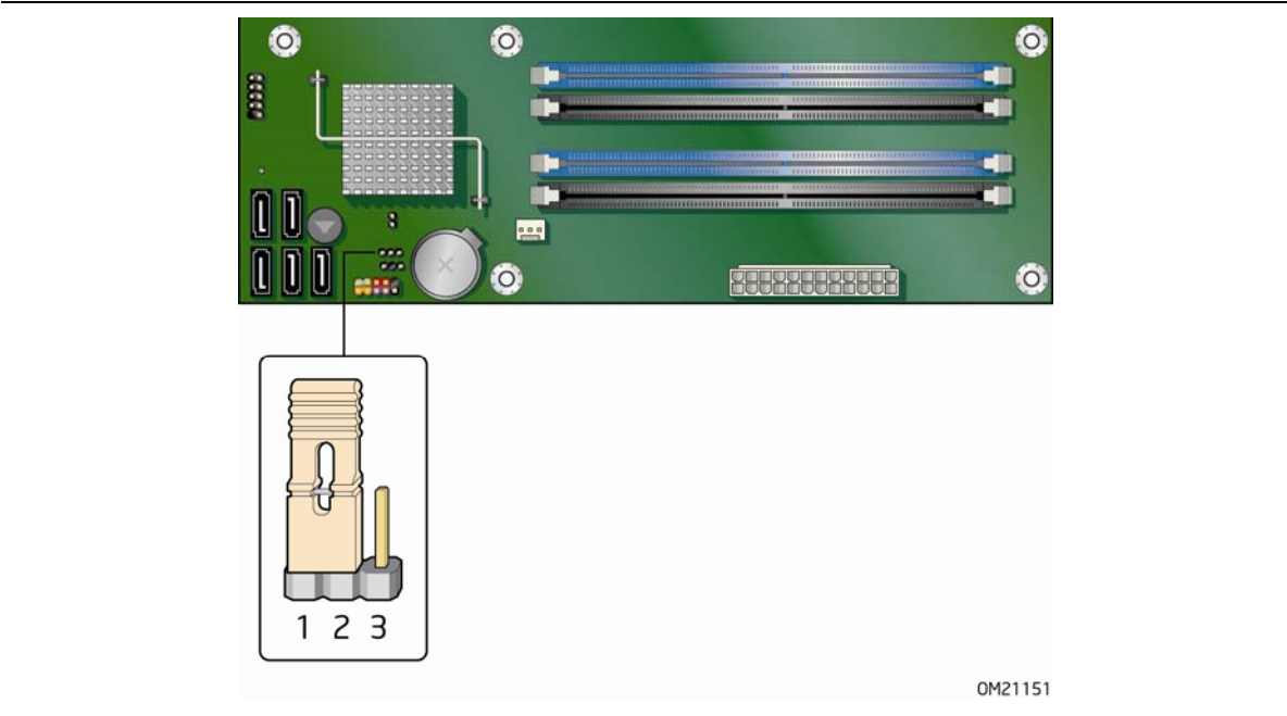
图 26. BIOS 配置跳线块位置
