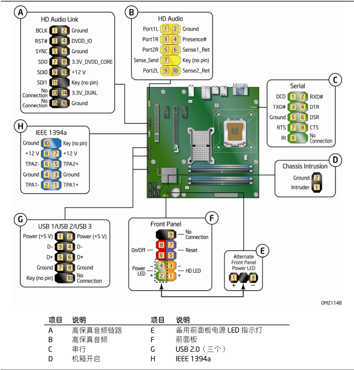
图 22. 内置接头连接器
