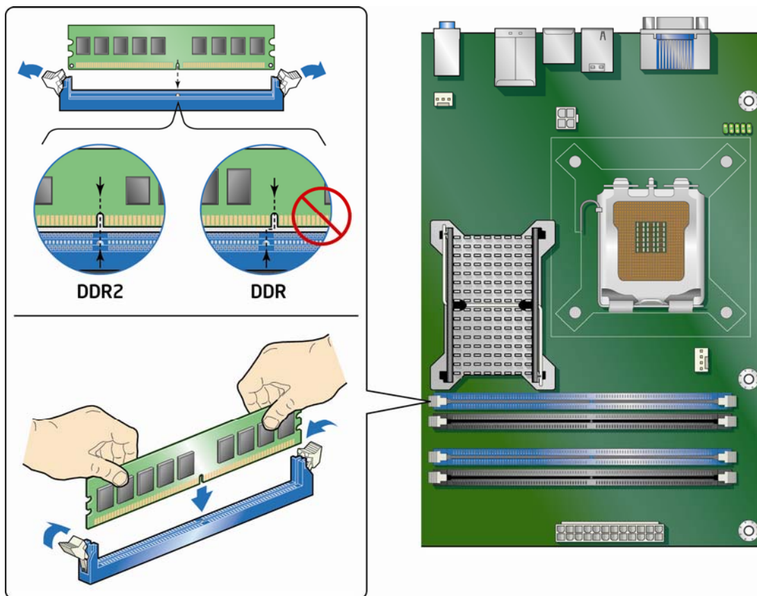
图 18. 安装 DIMM
