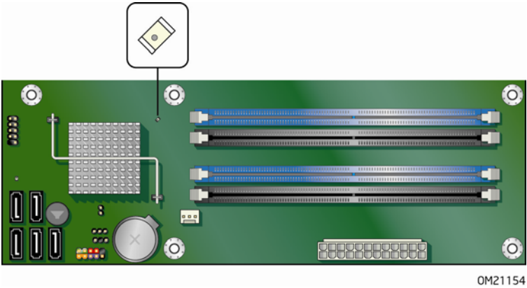
图 3. 英特尔 AMT 状态指示灯
