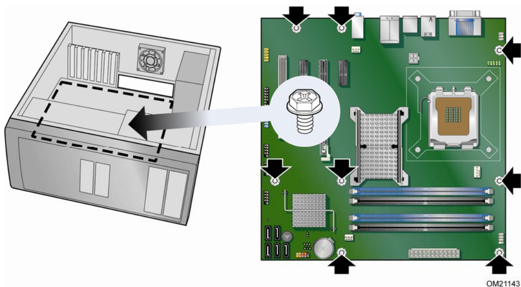
图 6. 英特尔台式机主板 DQ45CB 安装螺丝孔位置
