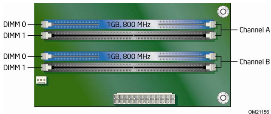
图 14. 两条 DIMM 双通道内存配置
