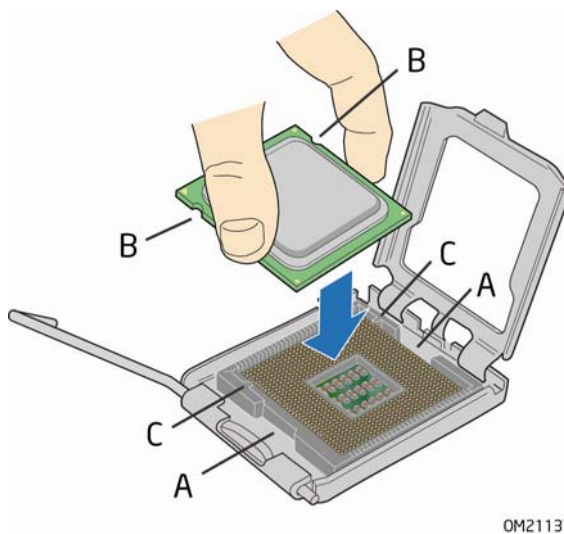
图 11. 安装处理器
