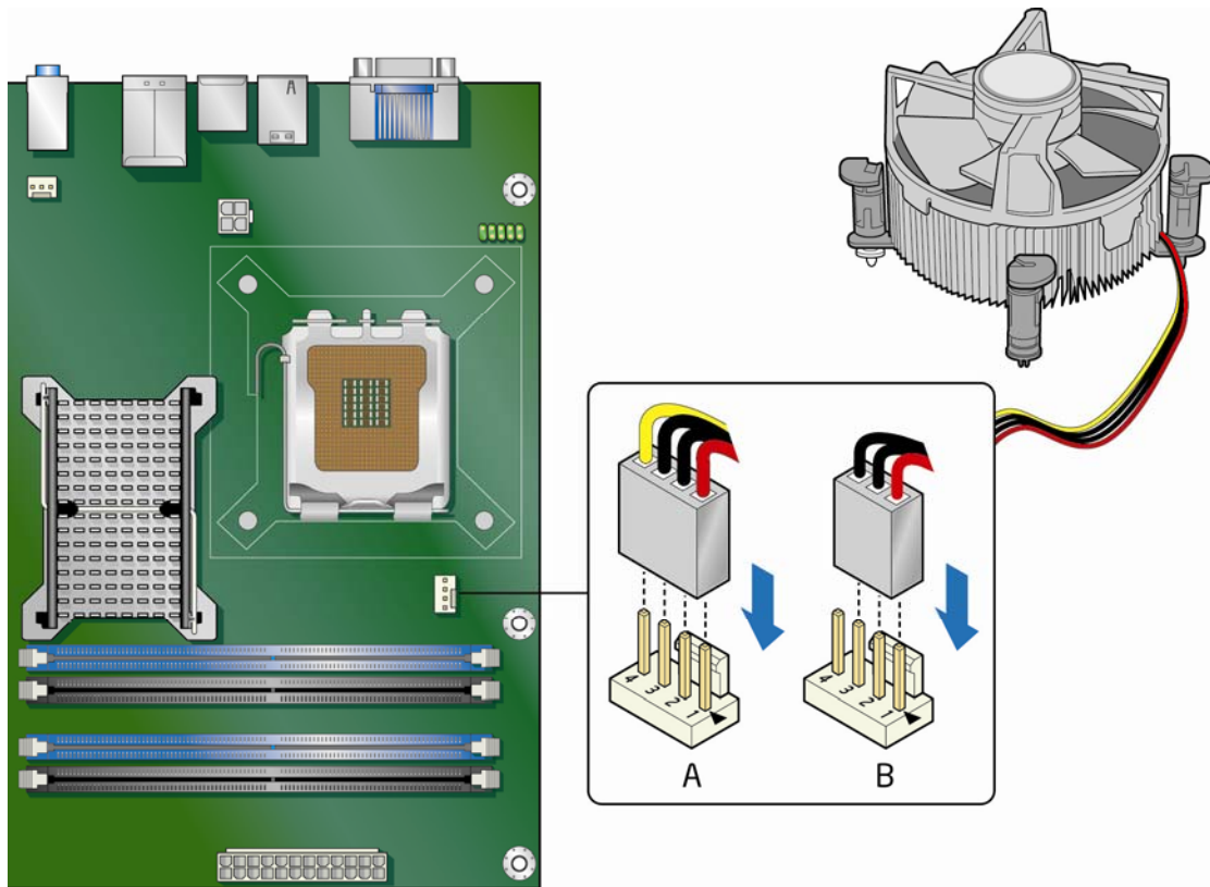
图 13. 连接处理器风扇散热器电缆
