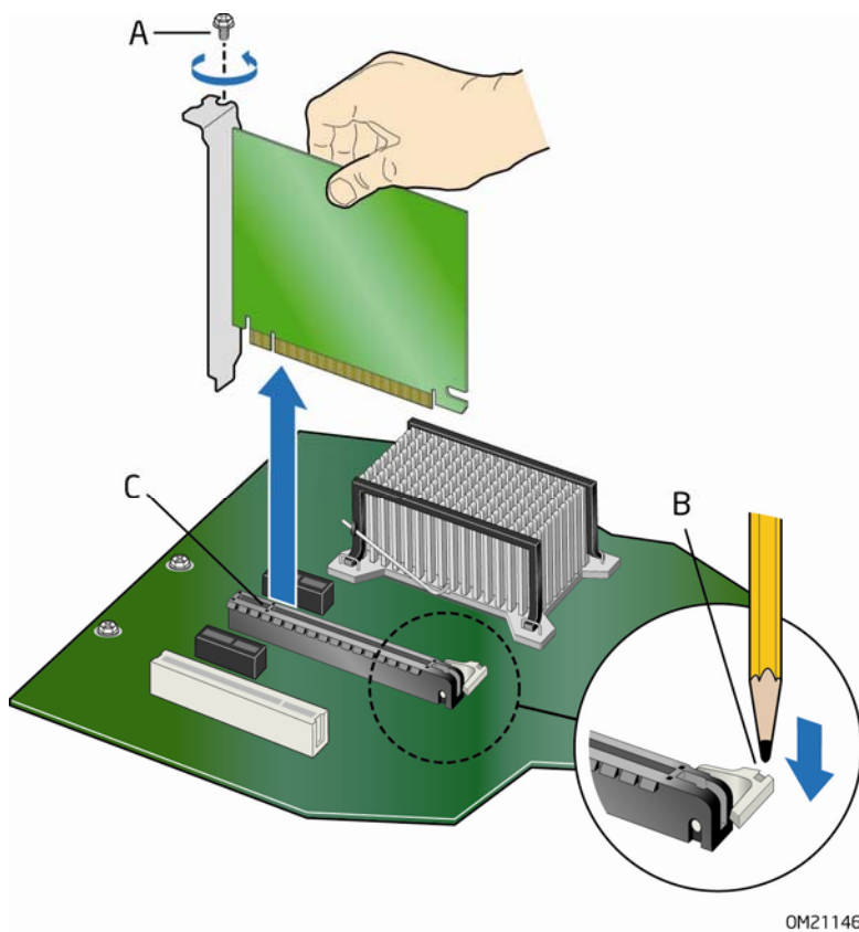
图 20. 拆卸 PCI Express x16 卡
