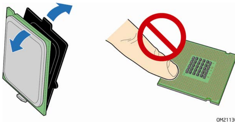
图 10. 从处理器保护罩中取出处理器
