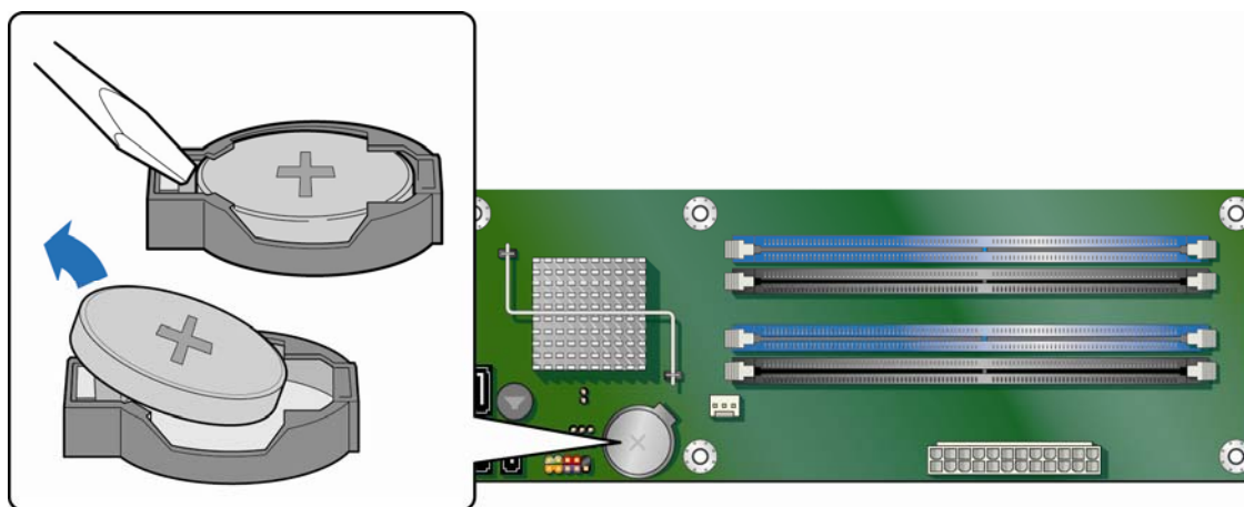
图 27. 拆卸电池
