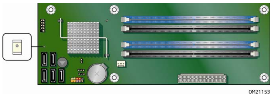
图 4. +5 V 备用电源指示灯位置
