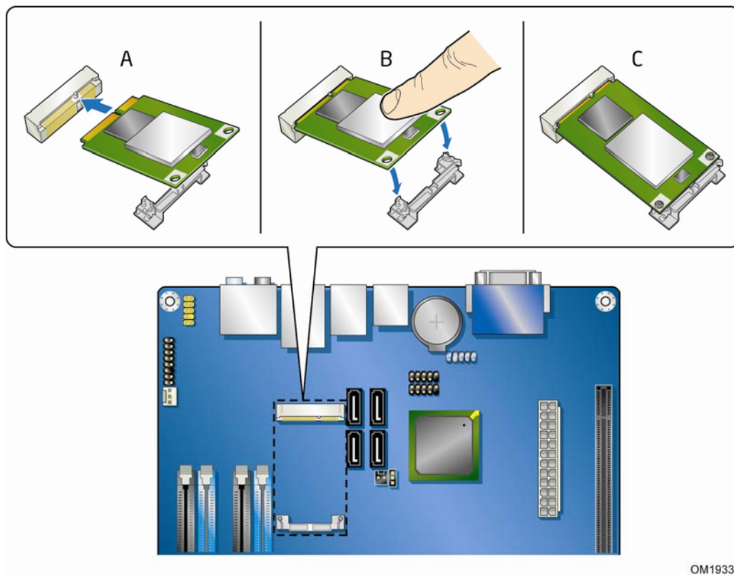
图 23. 安装 PCI Express Mini Card (PCI Express 微型卡)
