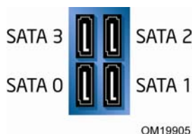
图 33. 台式机主板 DG965PZ 原始 SATA 端口映射
