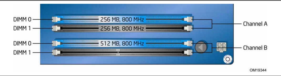
图 18. 双通道内存配置示例 3
