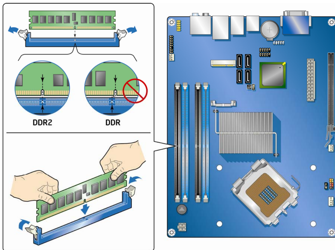
图 20. 安装 DIMM
