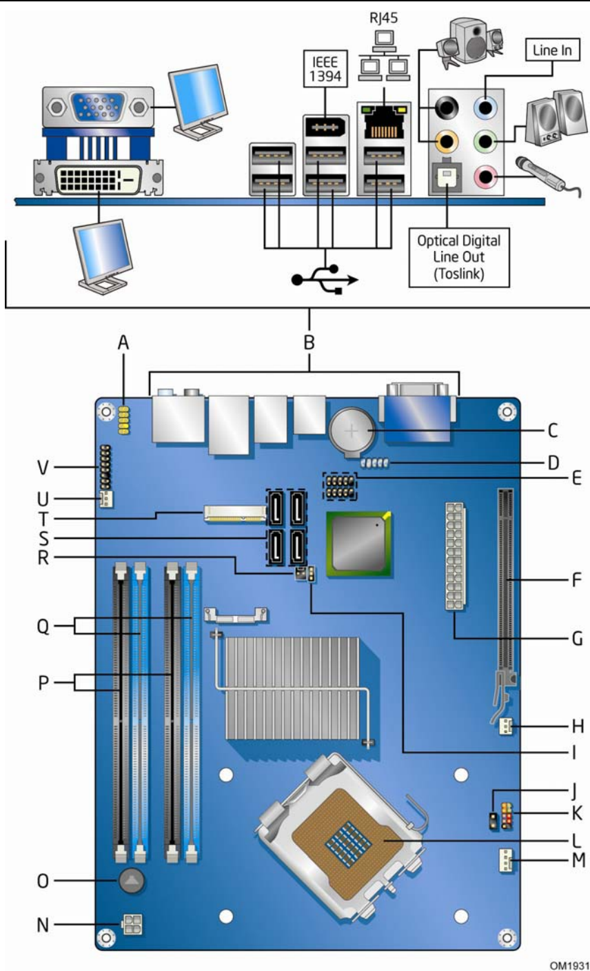
图 1. 台式机主板 DG965PZ 组件
