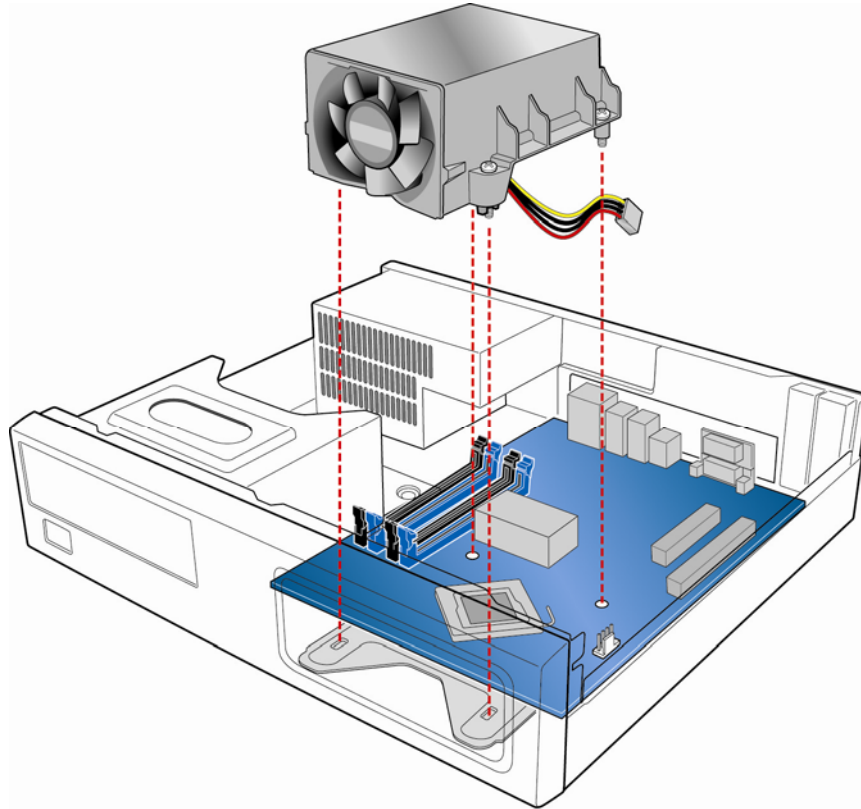
图 12. 散热模块相对于安装孔的位置
