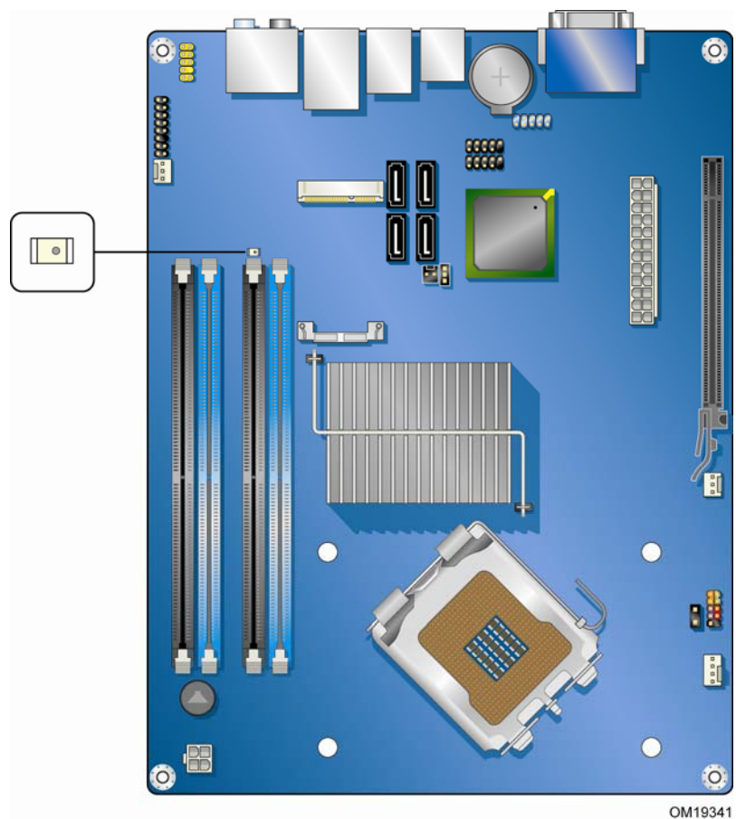
图 3. 备用电源指示灯位置
