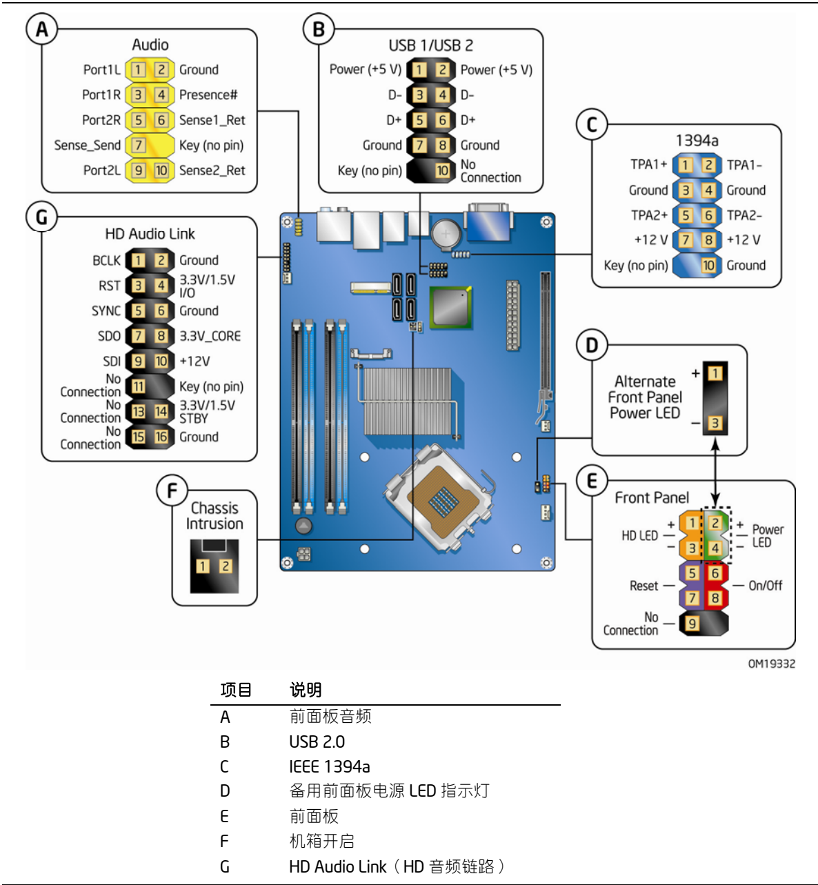
图 26. 内部接头连接器
