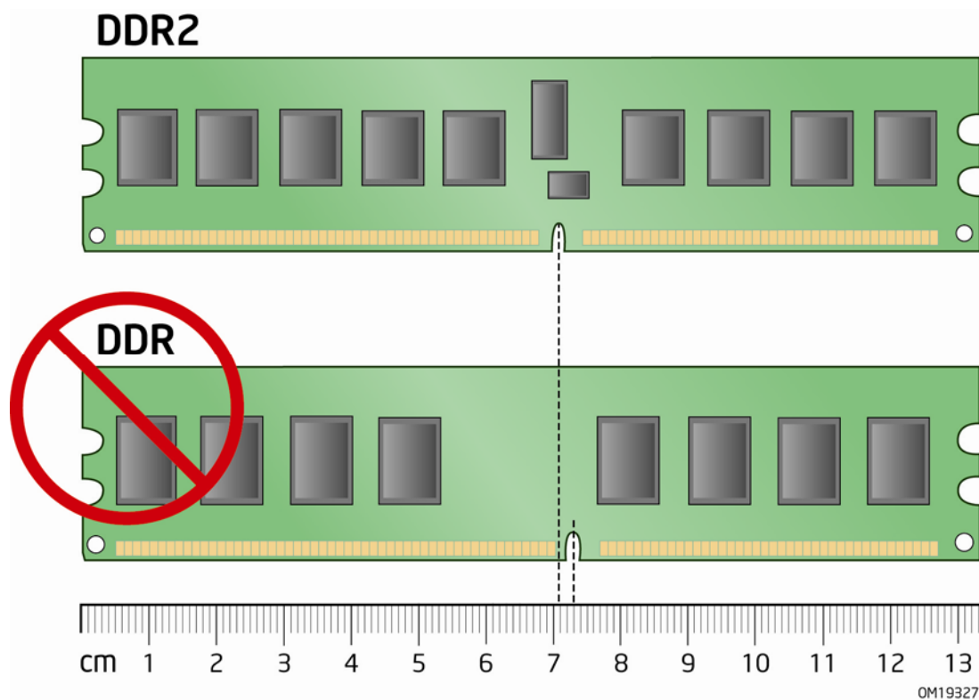
图 19. 使用 DDR2 DIMM
