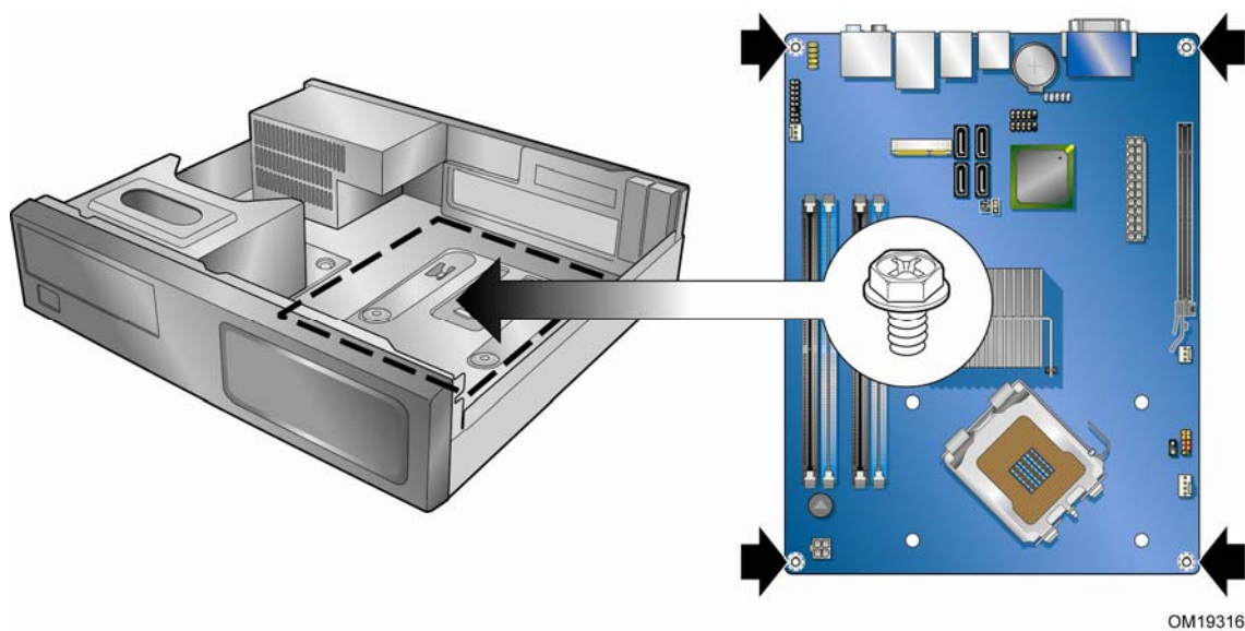
图 5. 台式机主板 DG965PZ 安装螺丝孔位置
