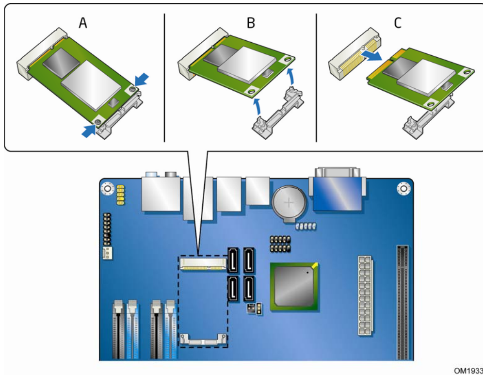
图 24. 拆卸 PCI Express Mini Card (PCI Express 微型卡)
