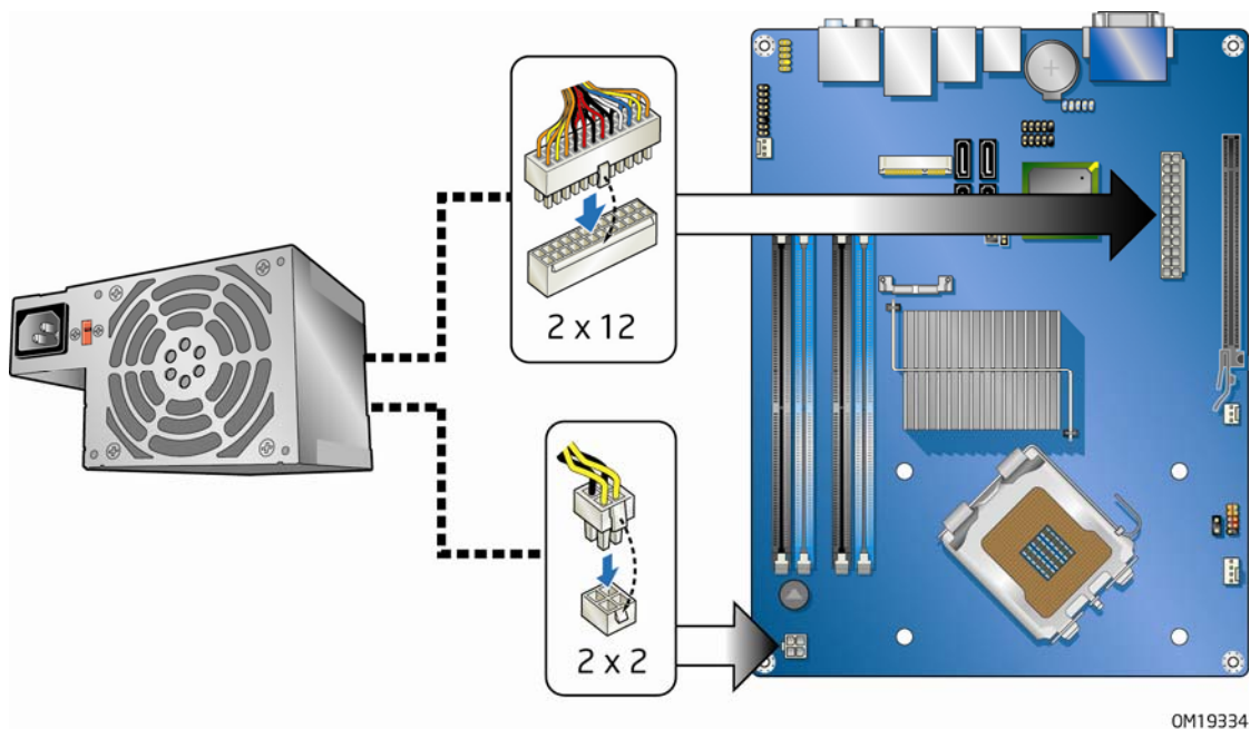
图 29. 连接电源系统电缆
