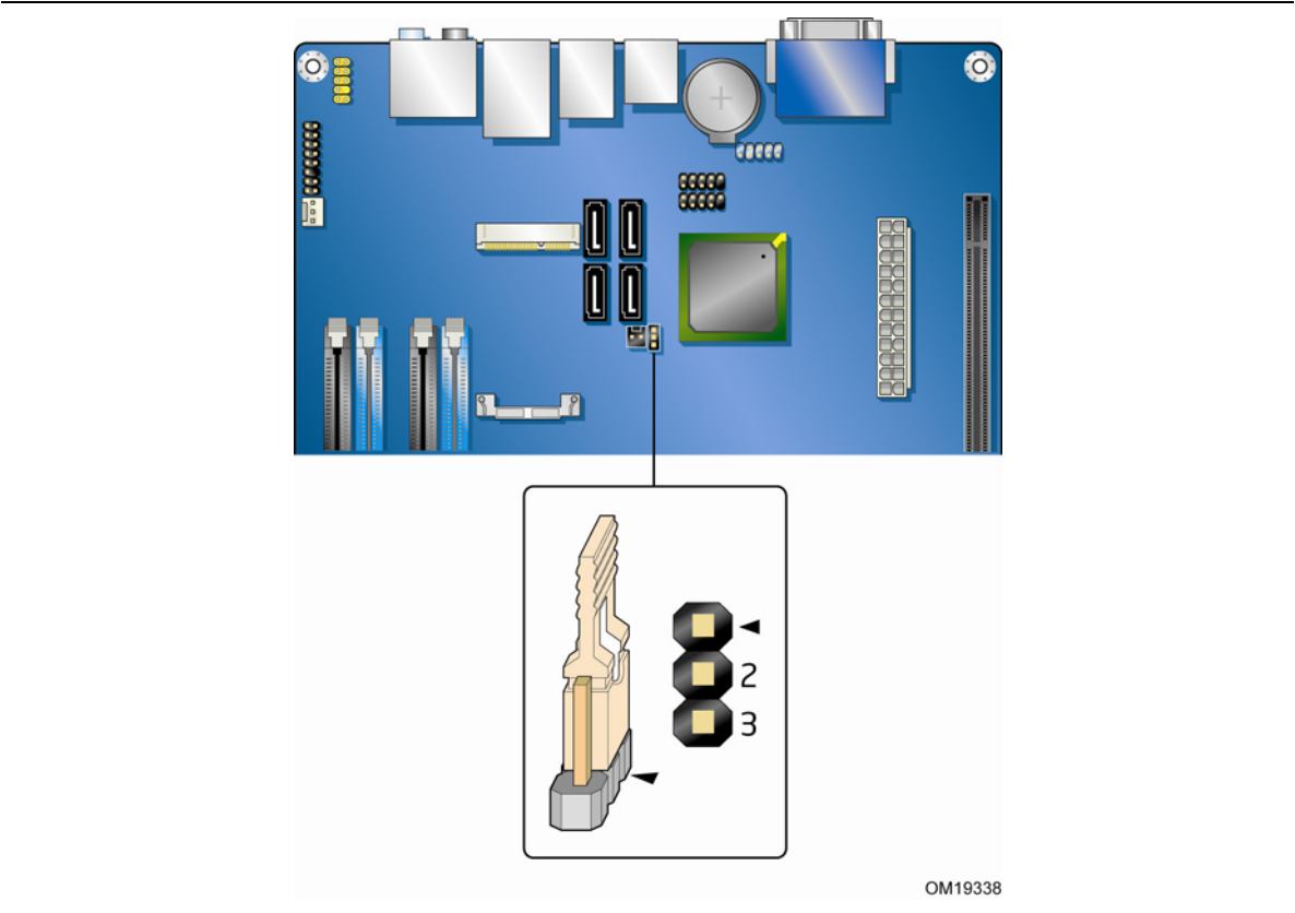
图 30. BIOS 配置跳线块位置
