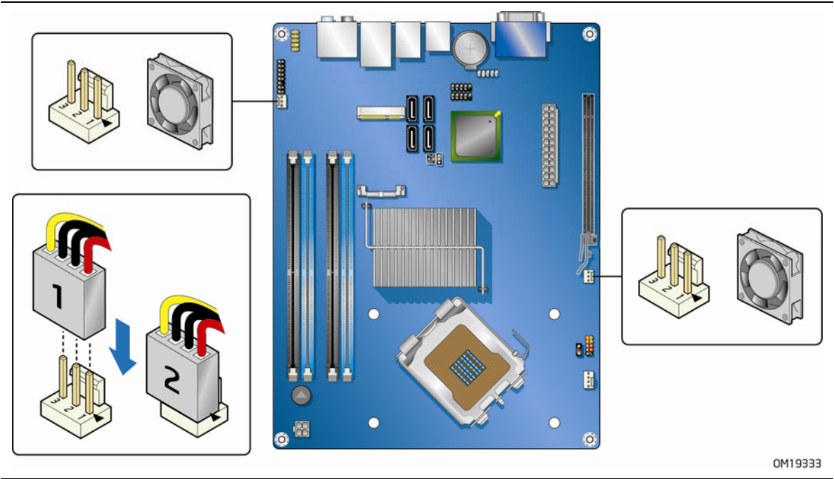
图 28. 机箱风扇接头连接器位置
