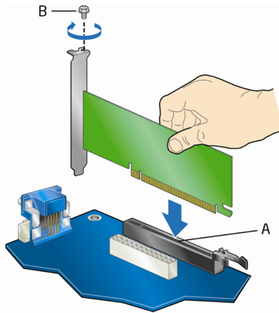
图 21. 安装 PCI Express x16 卡
