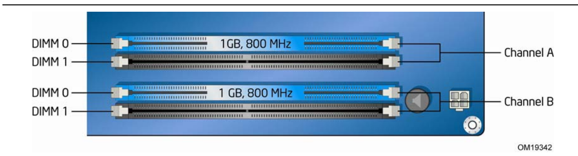
图 16. 双通道内存配置示例 1
