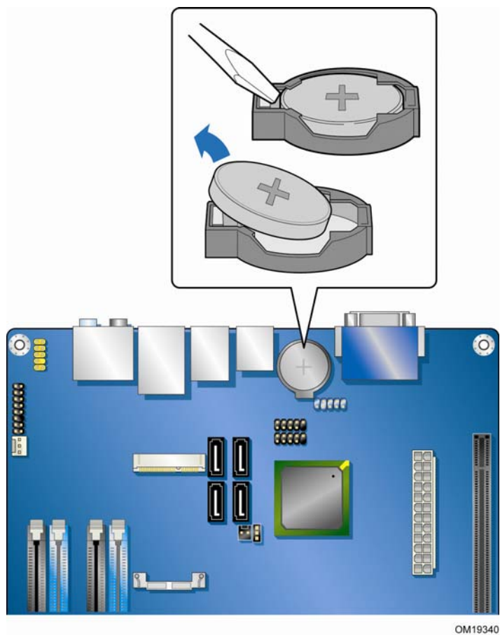
图 32. 拆卸电池
