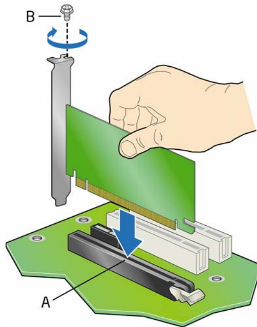
图 19. 安装 PCI Express x16 卡
