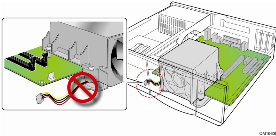
图 13. 小心温度模块风扇电缆的布线
