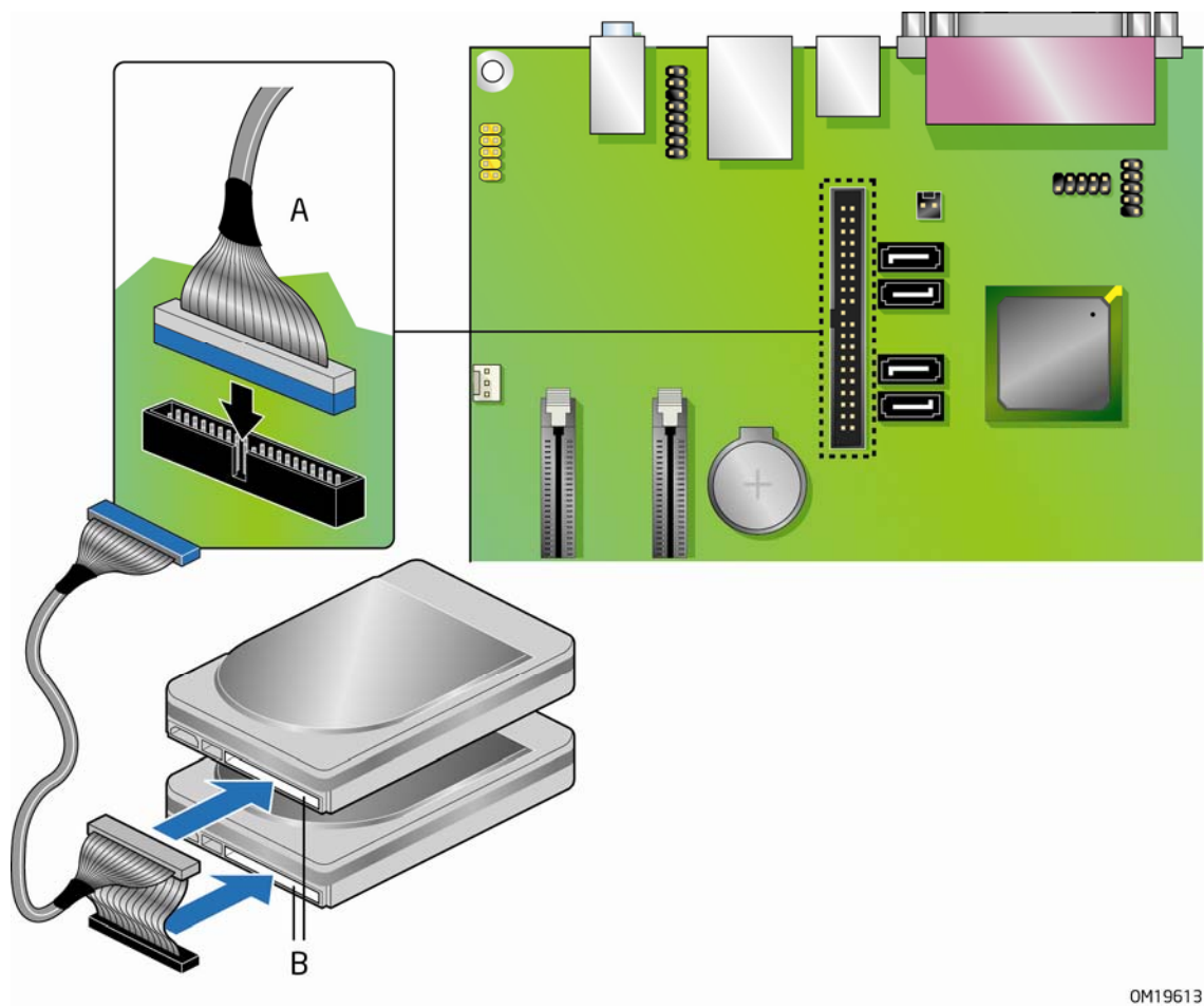
图 21. 连接 IDE 电缆
