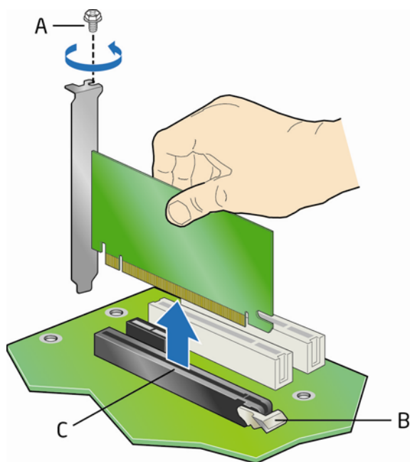
图 20. 拆卸 PCI Express x16 卡
