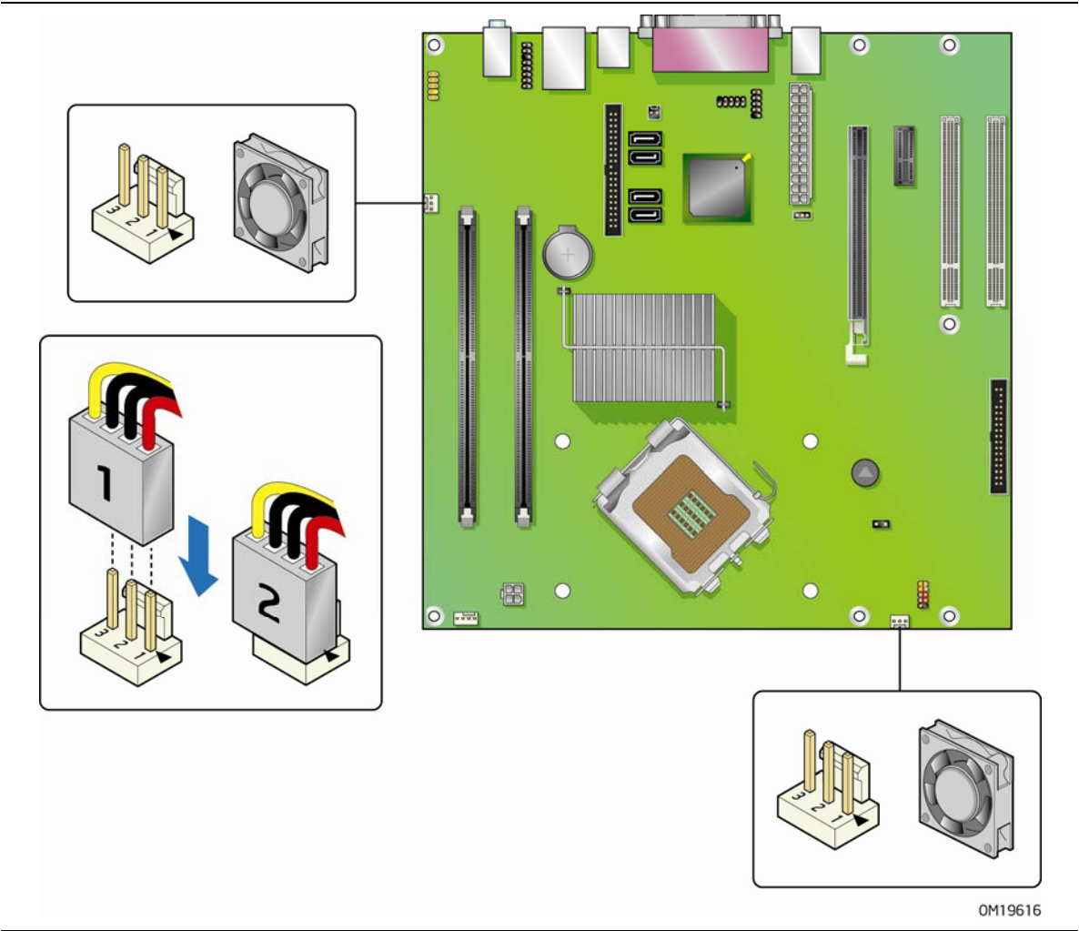
图 25. 机箱风扇接头连接器位置
