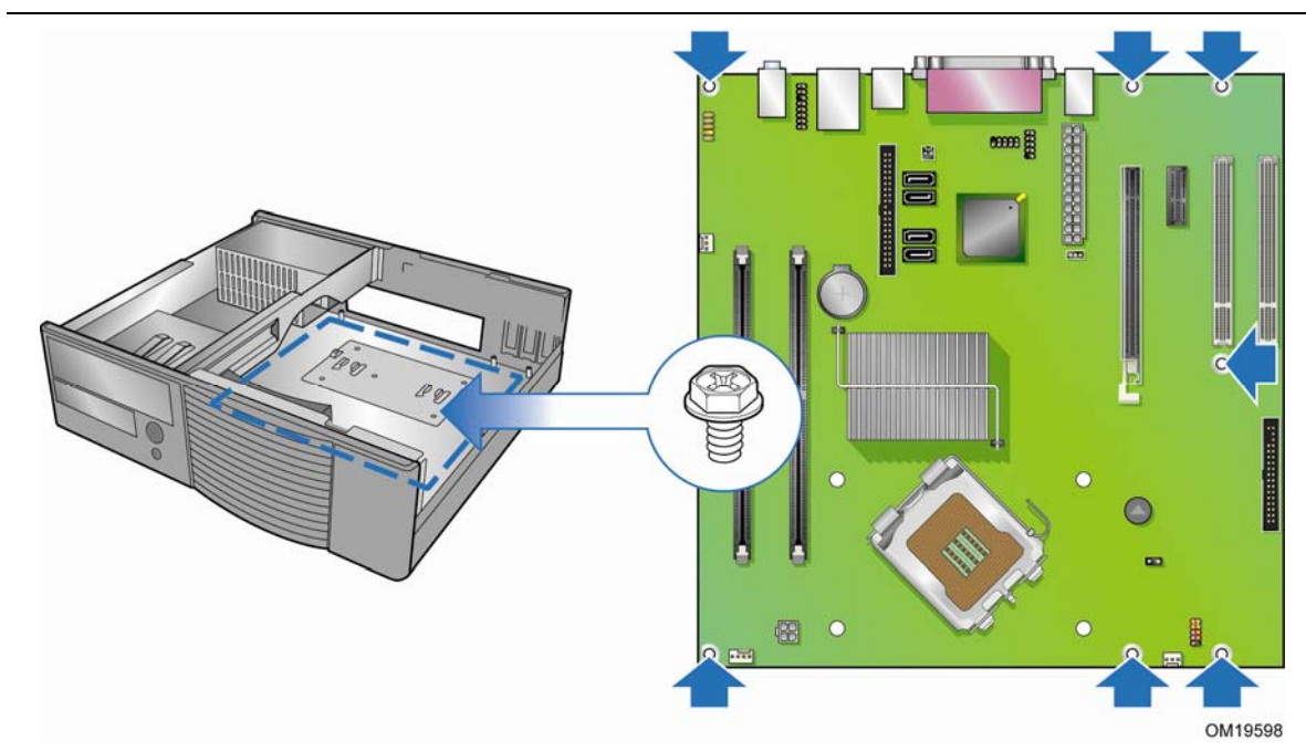
图 5. 台式机主板 D946GZTS 安装螺丝孔位置
