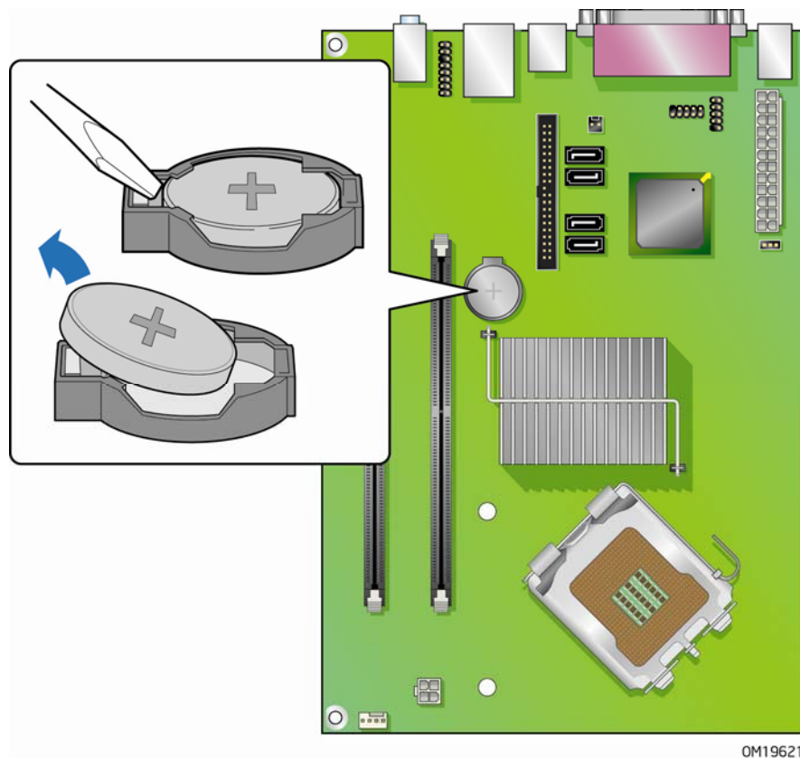
图 30. 拆卸电池
