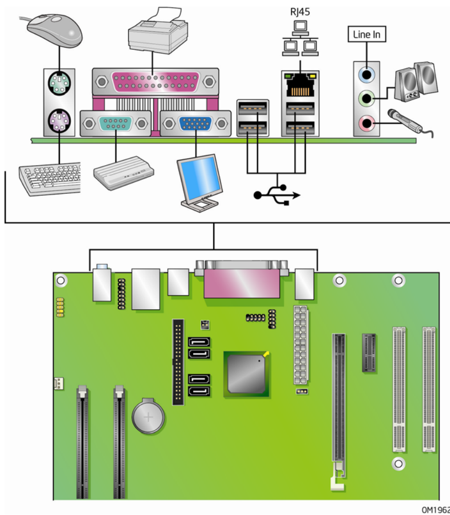
图 29. 背面板连接器
