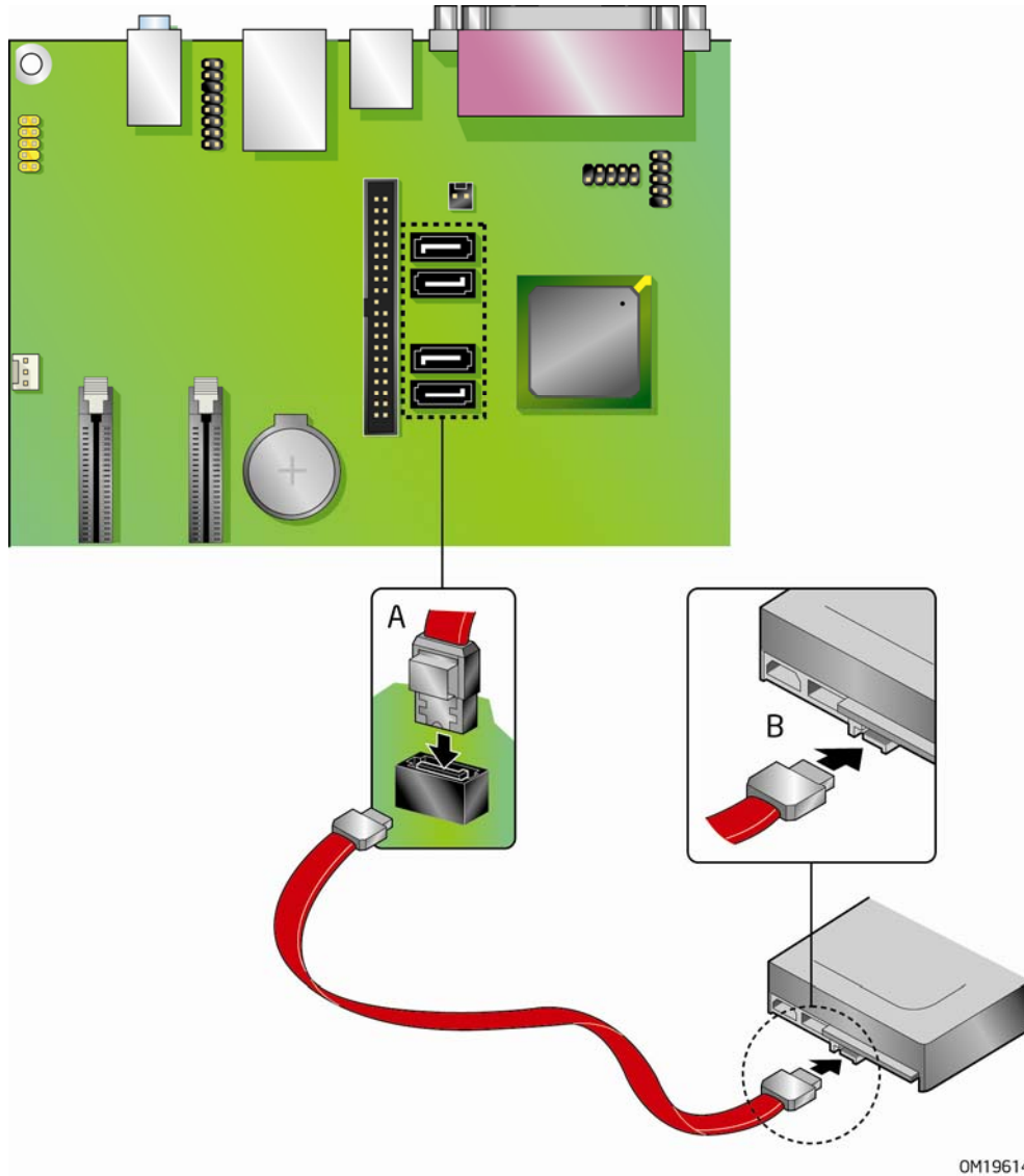
图 22. 连接串行 ATA 电缆
