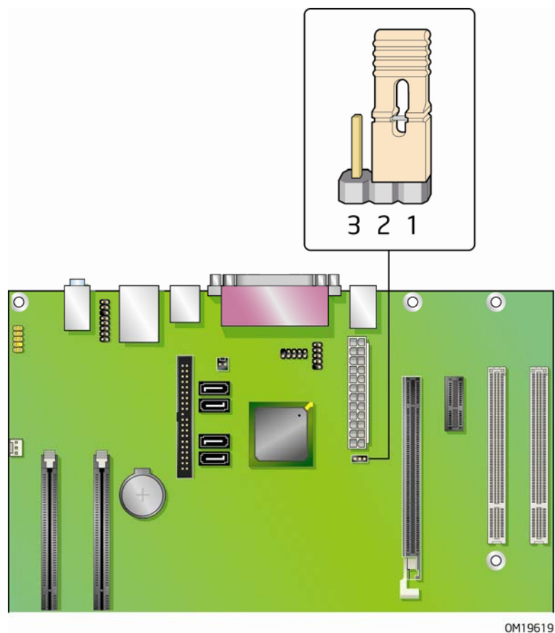
图 28. BIOS 配置跳线块位置
