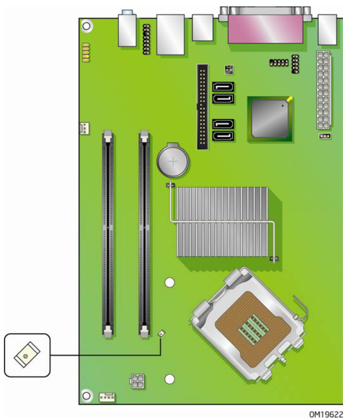
图 3. 备用电源指示灯位置
