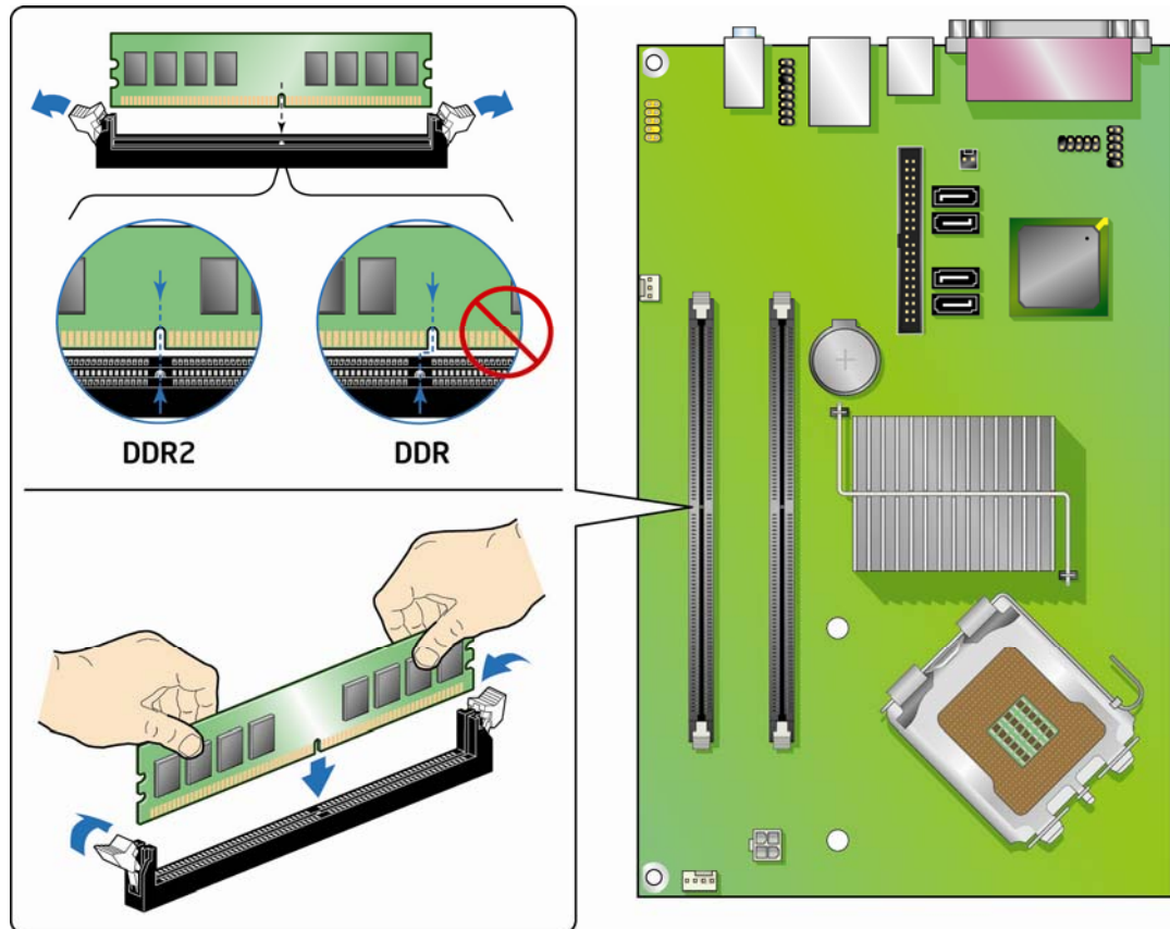
图 18. 安装 DIMM
