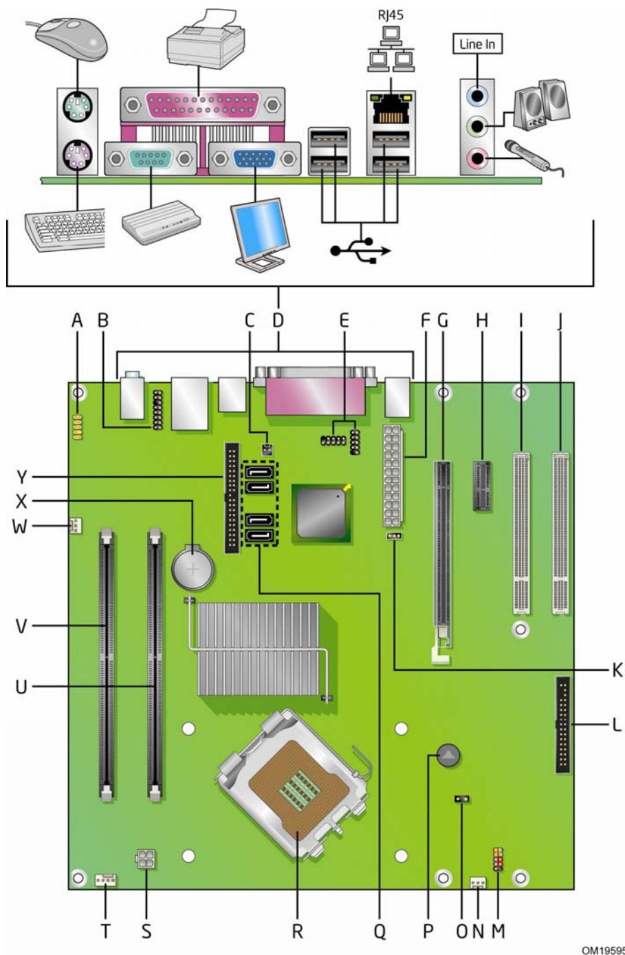
图 1. 台式机主板 D946GZTS 组件
