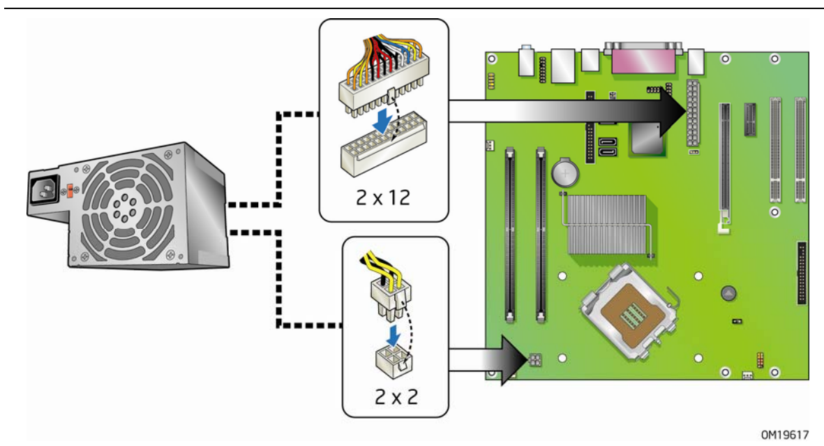
图 26. 连接电源系统电缆
