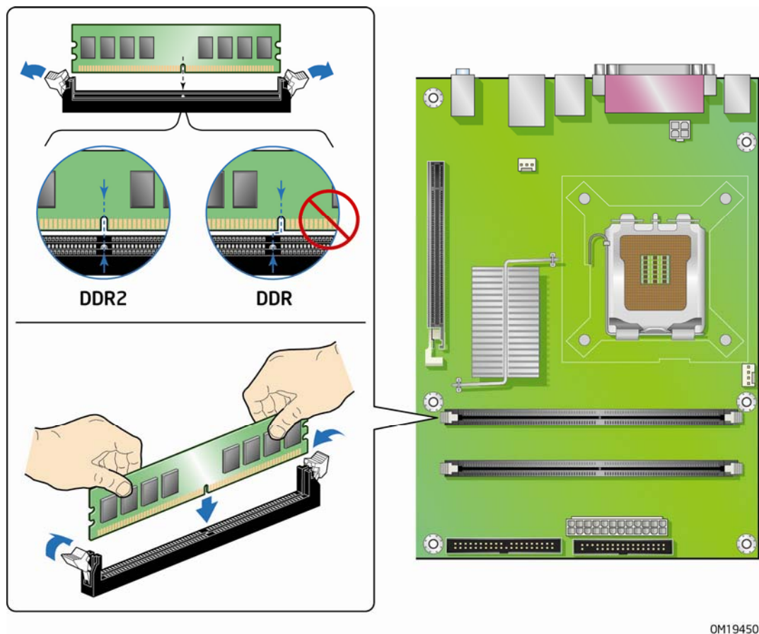
图 15. 安装 DIMM
