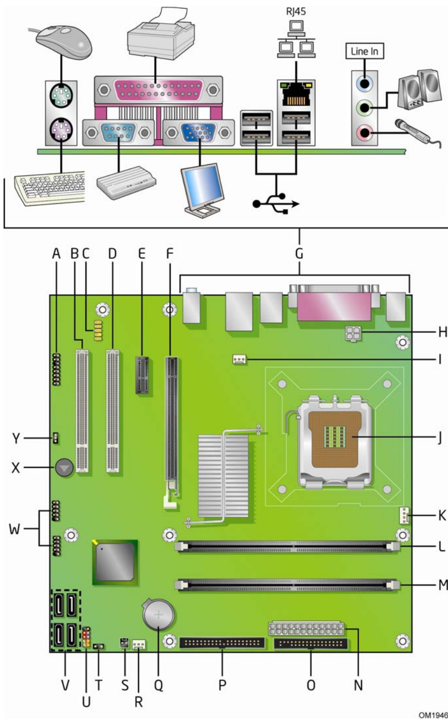
图 1. 台式机主板 D946GZIS 组件
