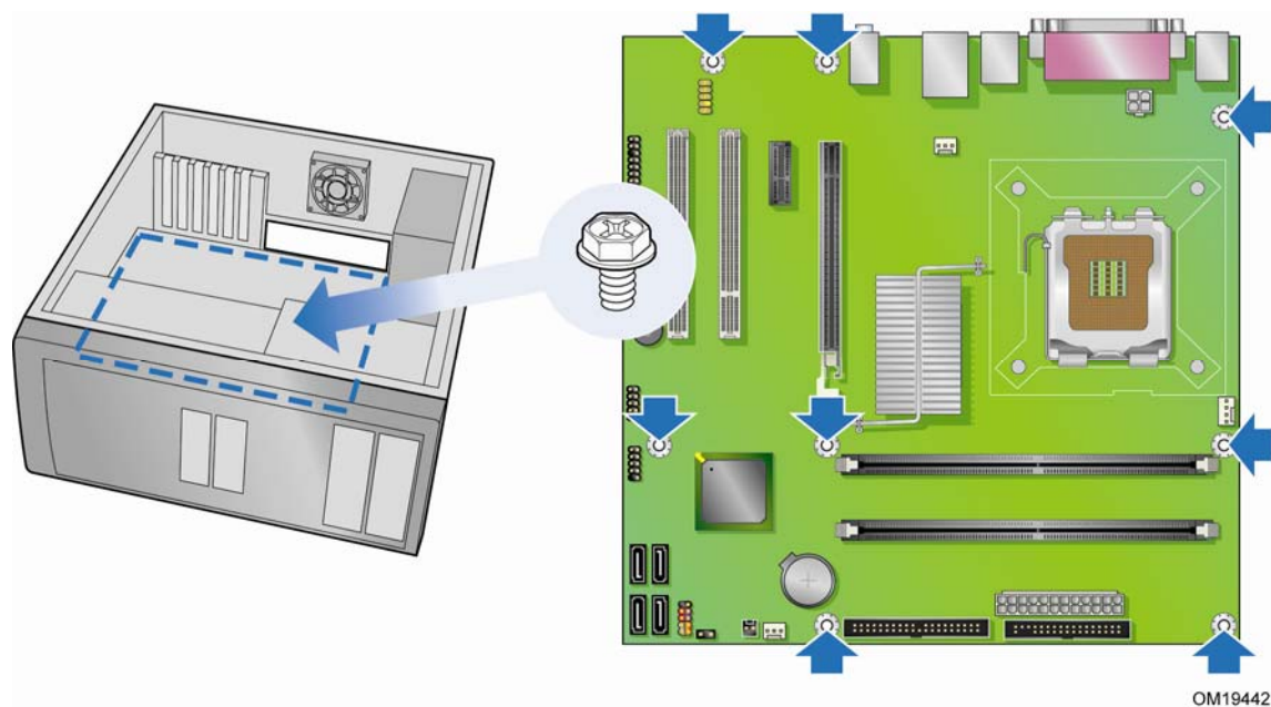
图 5. 台式机主板 D946GZIS 安装螺丝孔位置
