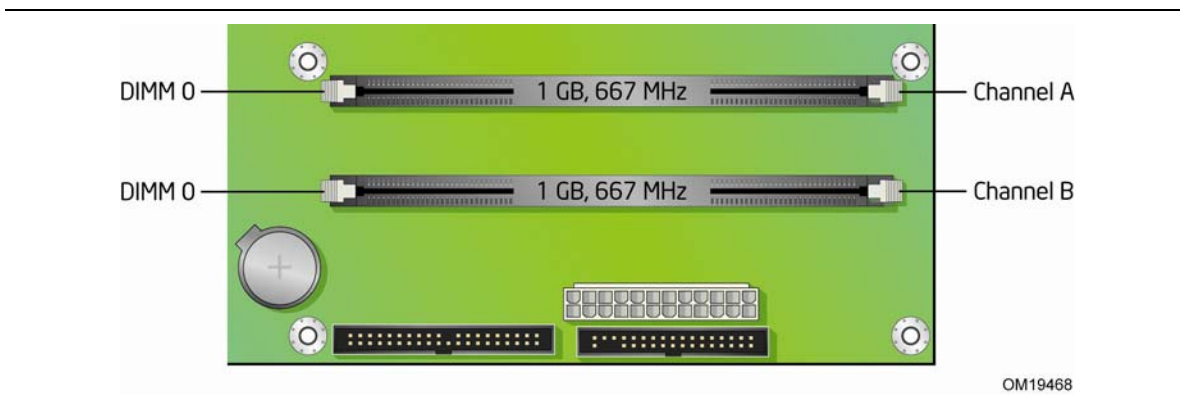
图 13. 双通道内存配置示例
