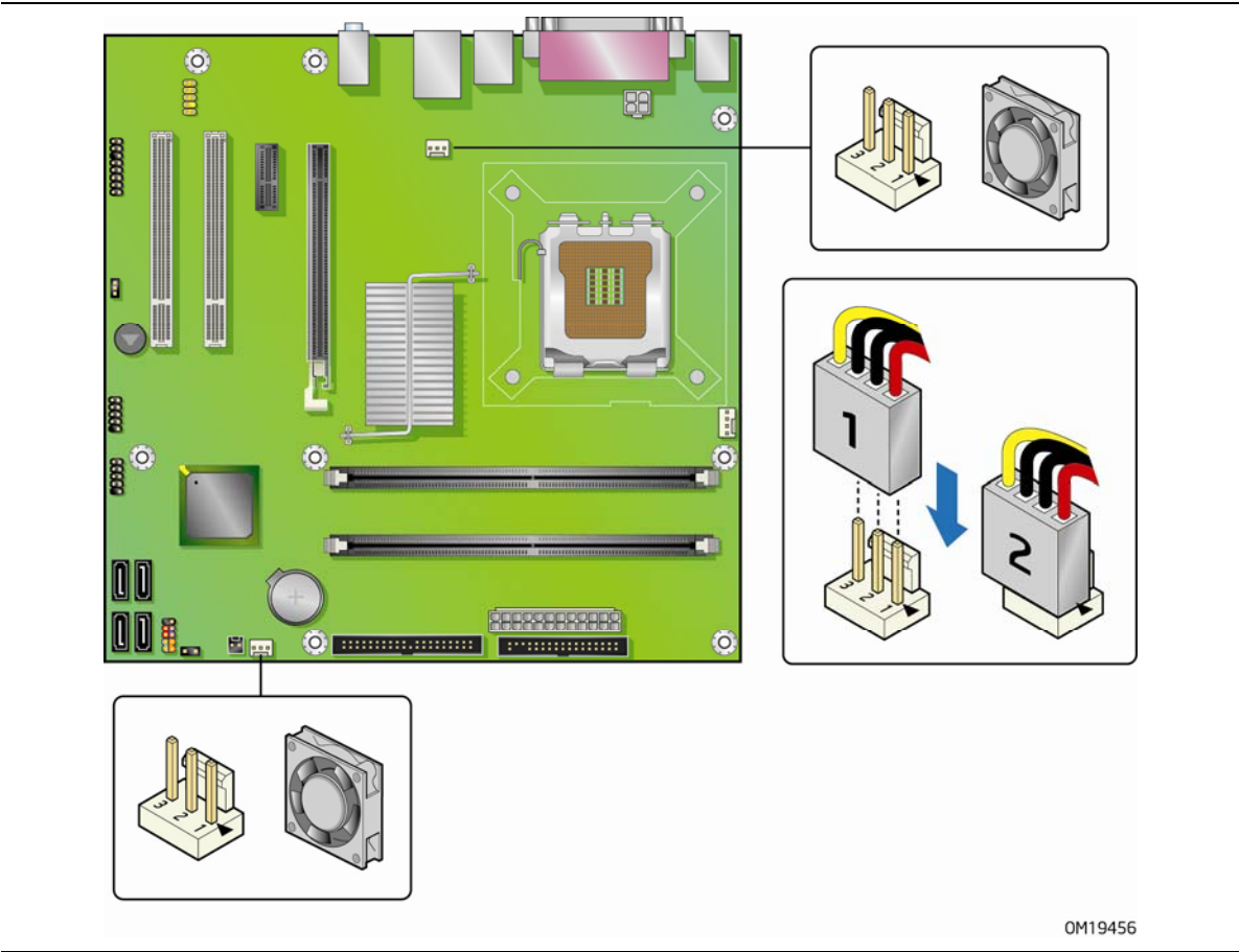
图 22. 机箱风扇接头连接器位置
