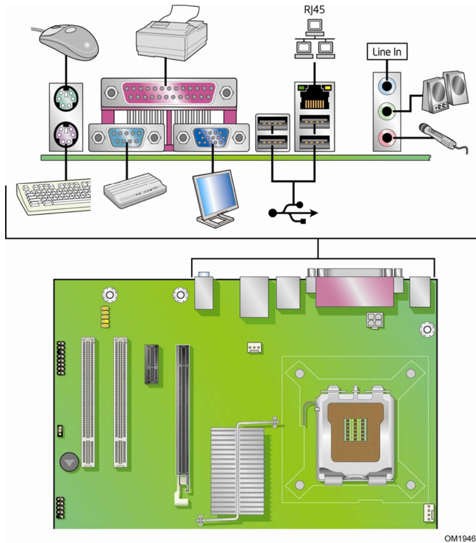
图 26. 背面板连接器
