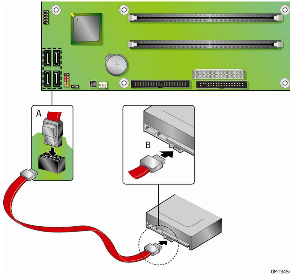
图 19. 连接串行 ATA 电缆
