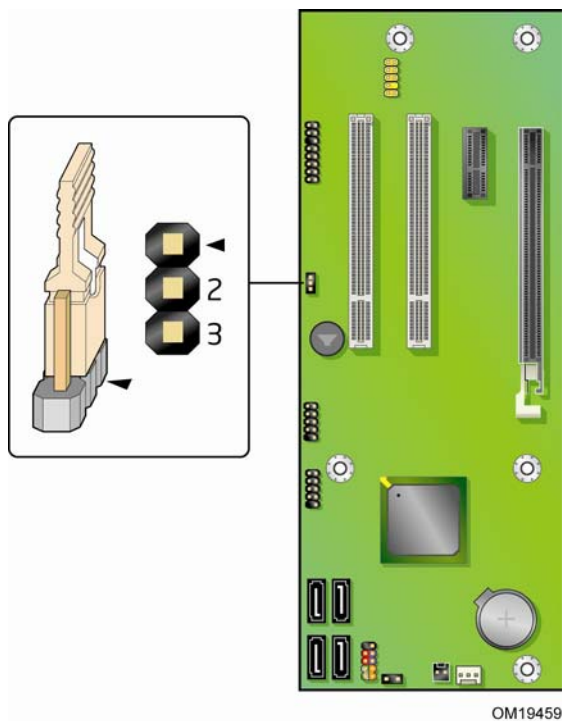
图 25. BIOS 配置跳线块位置
