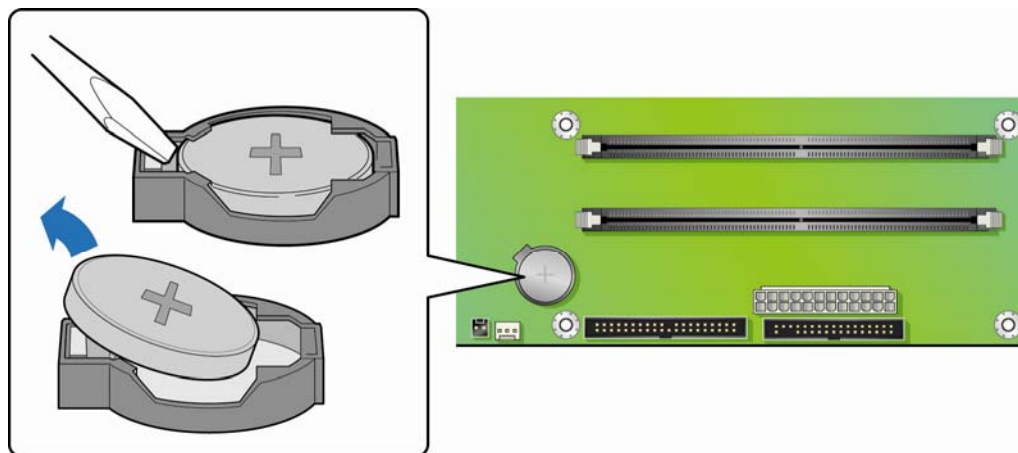
图 27. 拆卸电池
