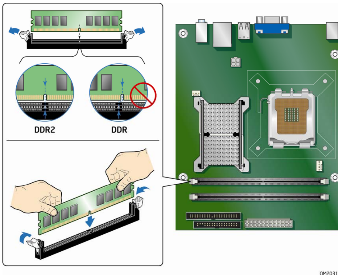
图 15. 安装 DIMM
