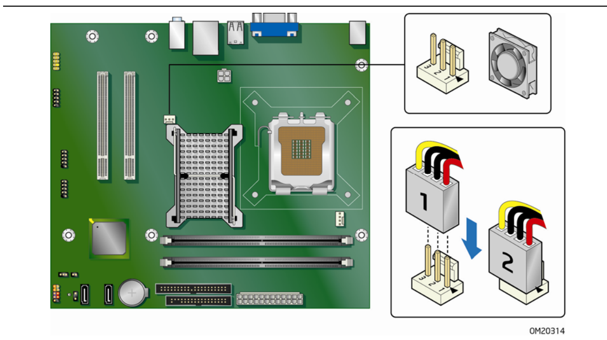
图 21. 机箱风扇接头连接器位置
