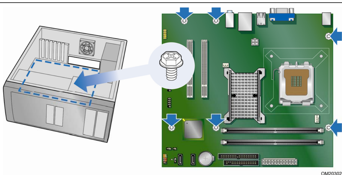
图 5. 台式机主板 D945GCPE 安装螺丝孔位置
