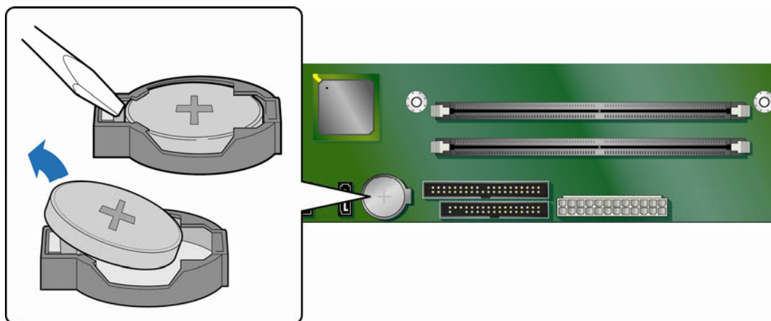
图 24. 拆卸电池
