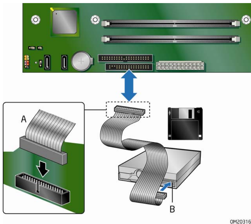
图 16. 连接软盘驱动器电缆
