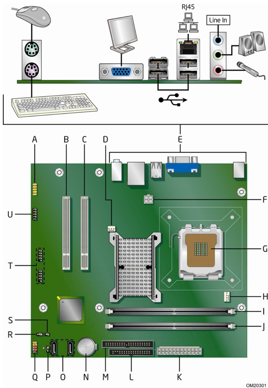
图 1. 台式机主板 D945GCPE 组件
