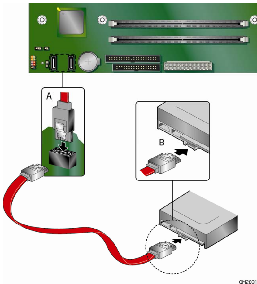
图 18. 连接串行 ATA 电缆
