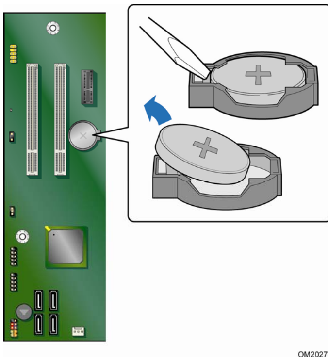
图 26. 拆卸电池
