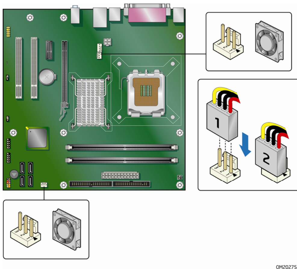
图 22. 机箱风扇接头连接器位置
