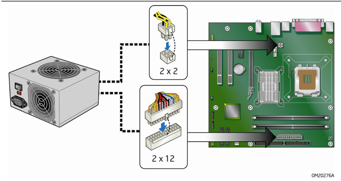
图 23. 连接电源系统电缆
