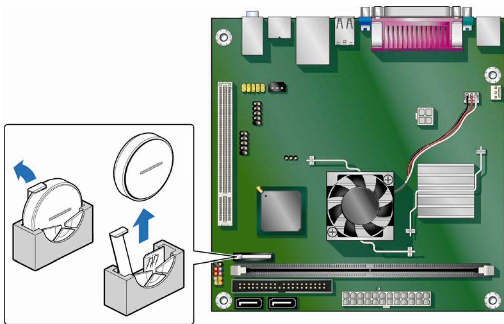
图 15. 拆卸电池
