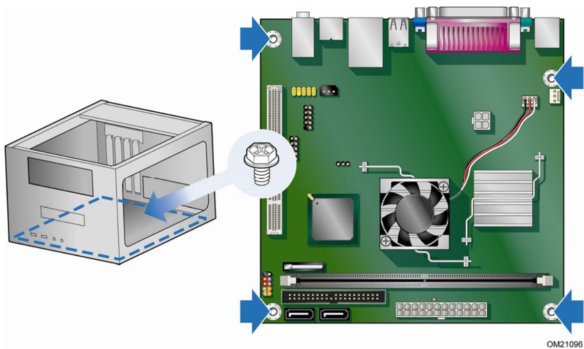
图 6. 英特尔台式机主板 D945GCLF2 安装螺丝孔
