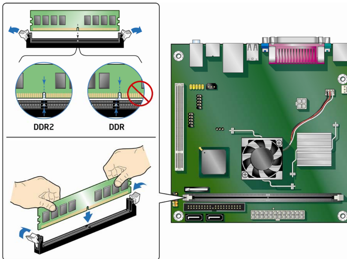
图 8. 安装 DIMM
