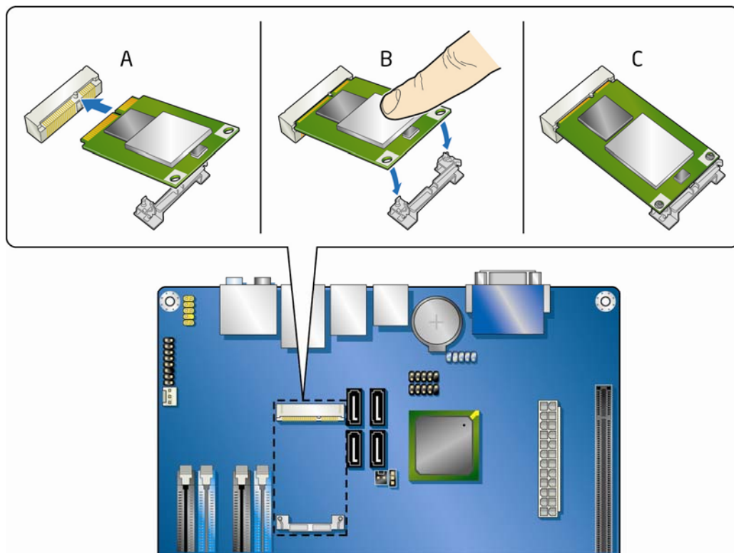
Figure 23. Installing a PCI Express Mini Card
