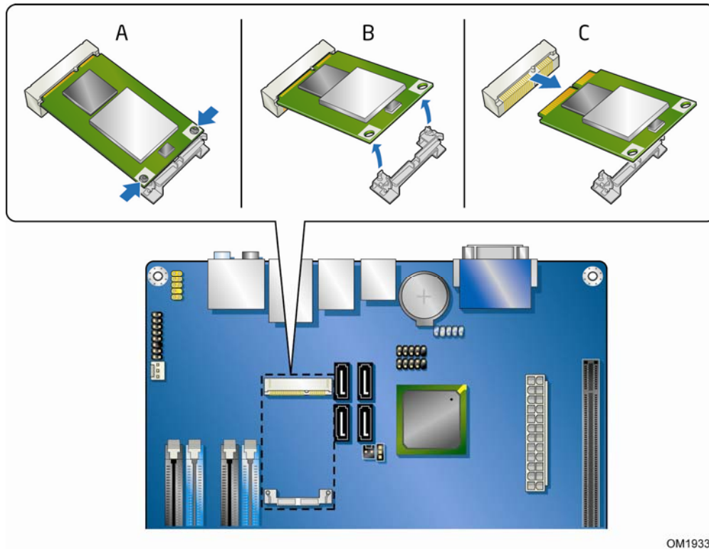
Figure 24. Removing a PCI Express Mini Card
