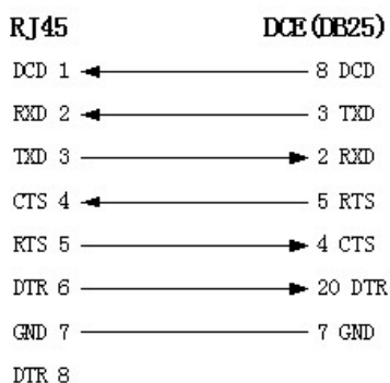
图 2-14. RJ45 与 DB25（DCE）连线图
