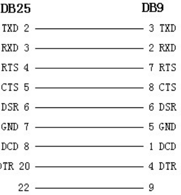
图 2-13 DB25 与 DB9 连线图
