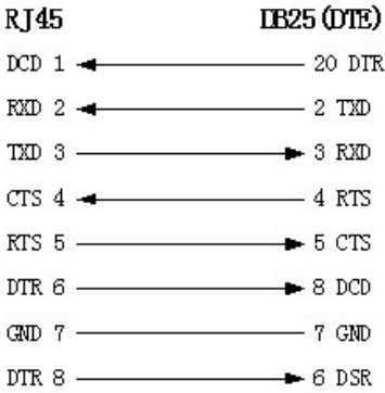
图 2-11. RJ45 与 DB25（DTE）连线图
