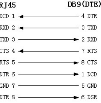
图 2-12. RJ45 与 DB9 连线图
