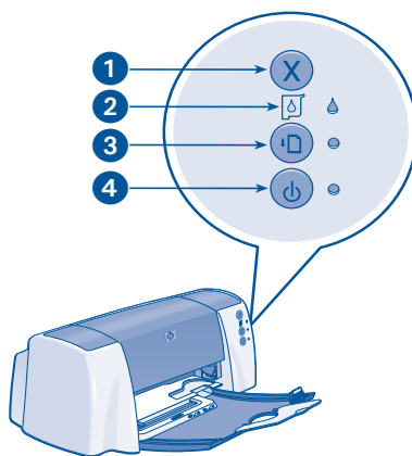
1. 取消按钮 2. 打印墨盒状态符号和指示灯 3. 继续按钮和指示灯 4. 电源按钮和指示灯
