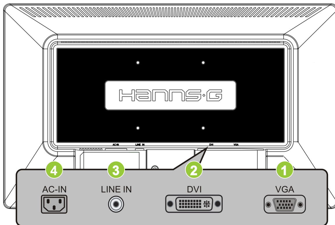
图二. 连接到 PC
