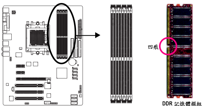
圖 1. 記憶體模組有一個凹痕，所以只能以一個方向插入。請扳開記憶體模組插槽卡榫，以雙手按在記憶體模組上邊兩側，以垂直向下平均施力的方式，將記憶體模組下壓推入插槽。
