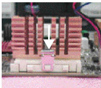
3. 先將CPU散熱風扇一邊的卡桿以平均施力的方式往下壓，直至扣緊為止以同樣地方式再將另一邊卡桿扣緊。
