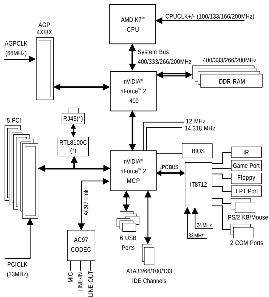
晶片組功能方塊圖 - GA-7N400E(-L)
