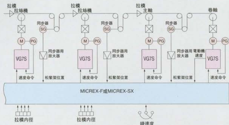
■控制框圖
