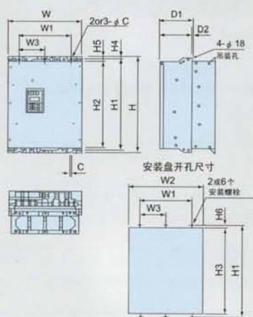
圖 D (外部冷卻方式)
