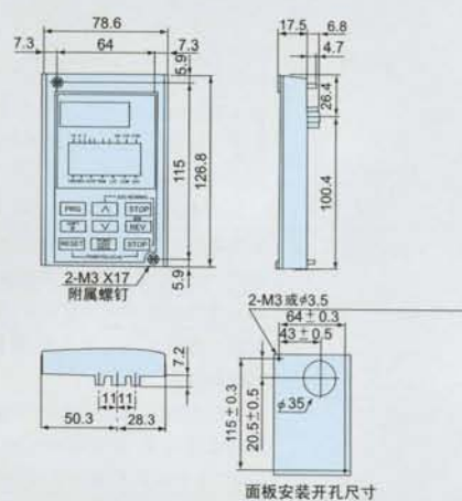
鍵盤顯示面板 (全機種通用)
