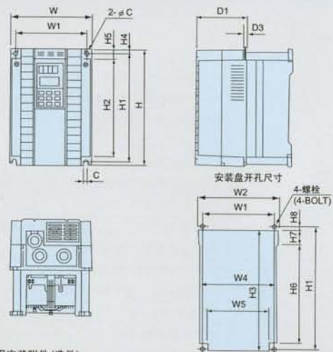
圖 B (外部冷卻方式)
