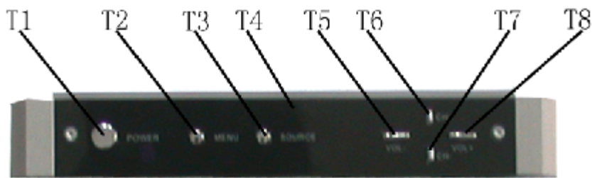
电视接收盒前视图
