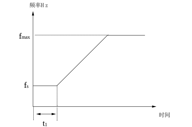
图6-26 起动频率与起动时间示意图
