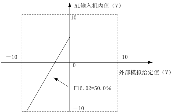
图6-76 高于零偏则等于零偏校正模式
