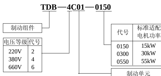
图2-7 制动单元型号说明
