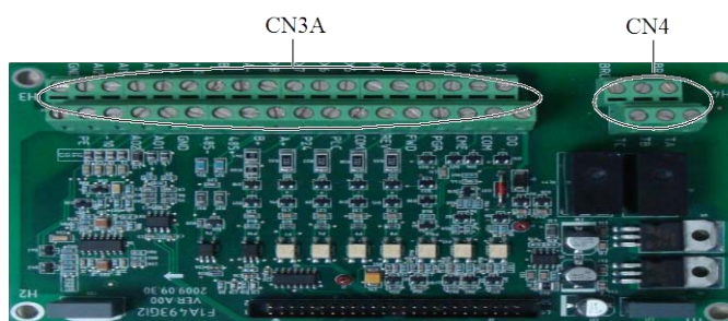
图4-7 控制回路端子在接口板上的位置示意图
