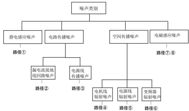
图4-35 噪声分类
