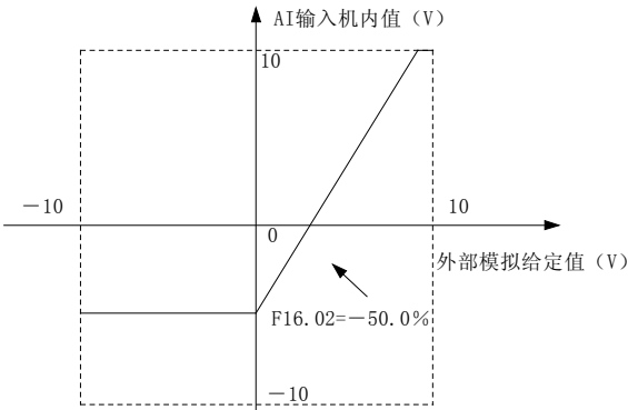
图6-75 低于零偏则等于零偏校正模式
