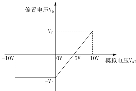
图6-70 输出电压偏置
