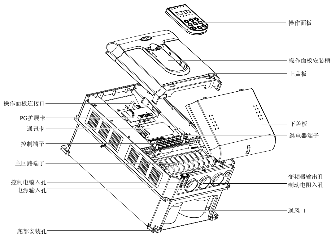
图2-1 22kW 及其功率等级以下变频器结构图
