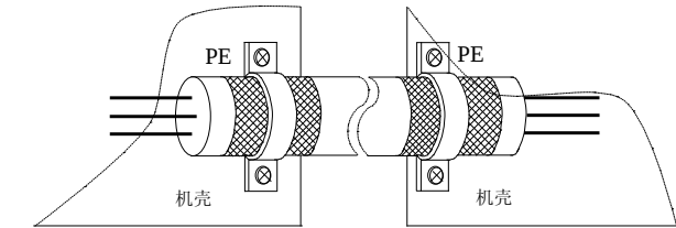
图4-38 正确的屏蔽接地方法
