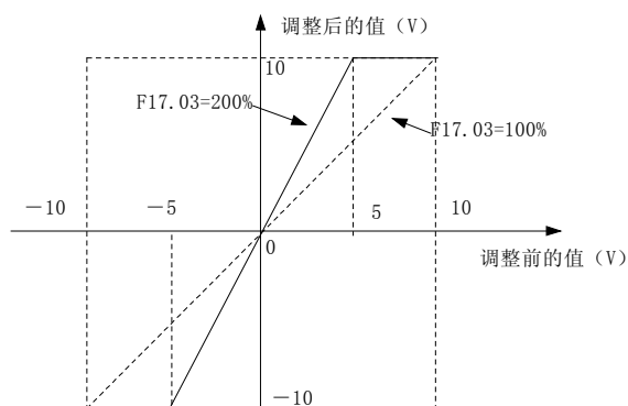
图6-79 模拟输出与增益关系曲线
