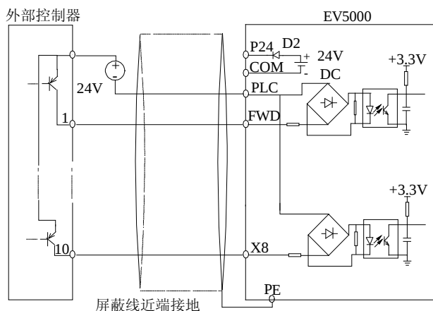
图4-26 使用外部电源的漏极连接方式
