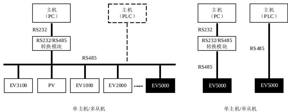
图8 变频器组网方式示意图
