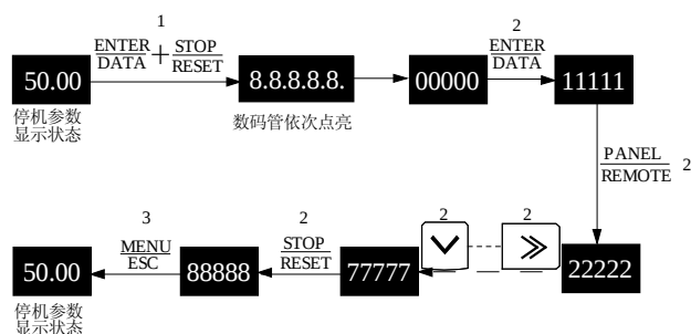
图5-3 LED 操作面板自检操作示例
