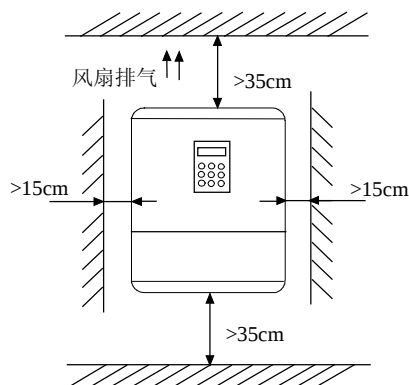
图3-2 安装的间隔距离（55kW 及以上）
