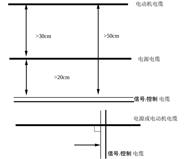
图4-37 系统配线要求
