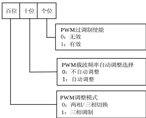
图6-35 PWM模式优化选择
