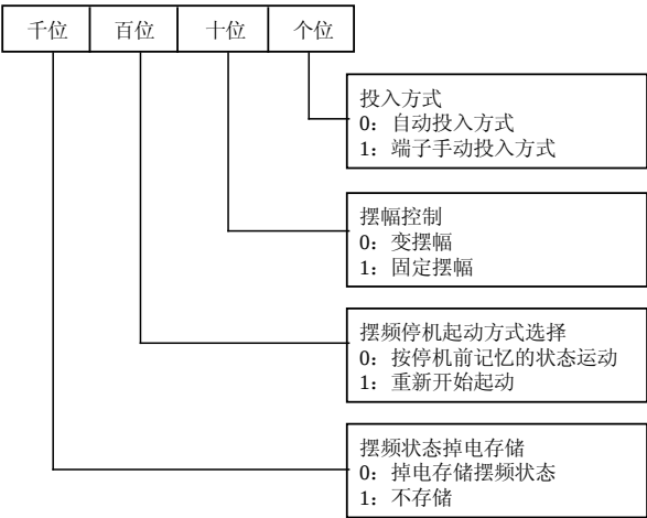
图6-96 摆频运行方式参数含义
