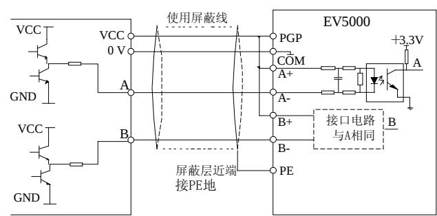
图4-32 推挽信号 PG 接线示意图
