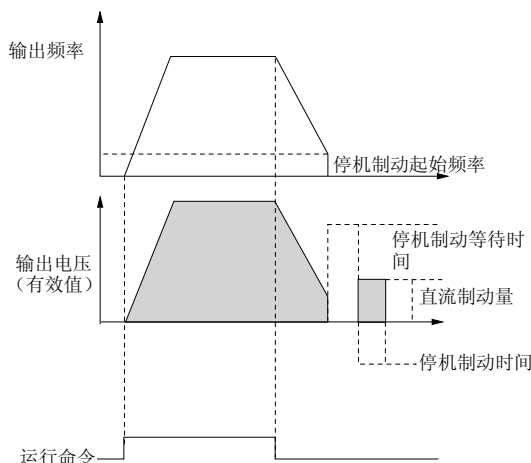
图6-28 减速停车+直流制动示意图
