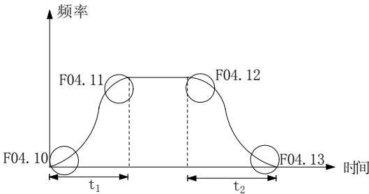
图6-19 加减速起始、结束时间说明
