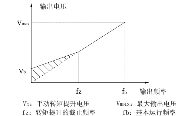
图6-94 转矩提升 (提升量为阴影部分)
