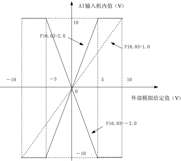
图6-72 模拟输入与增益关系曲线
