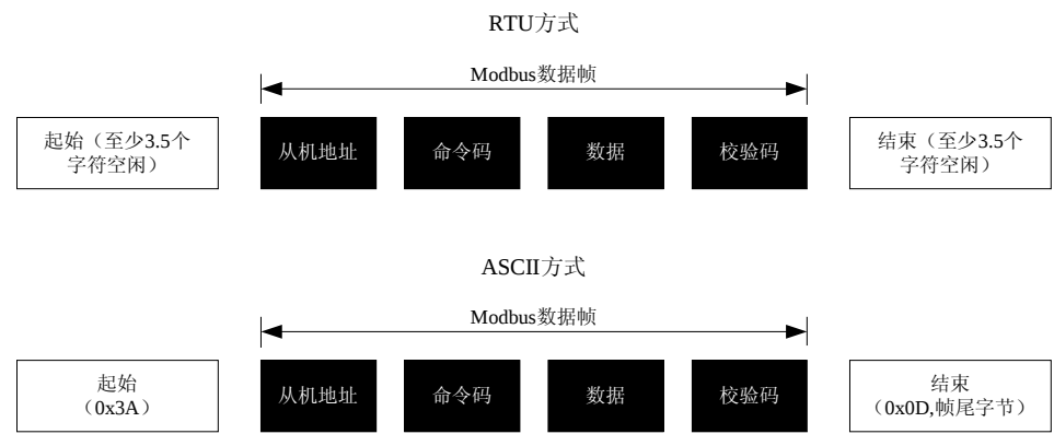
图9 Modbus 协议格式
