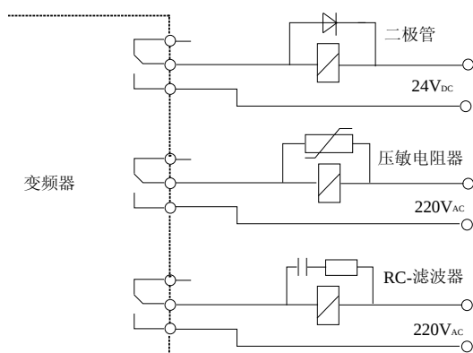
图4-44 继电器、接触器及电磁制动器要求
