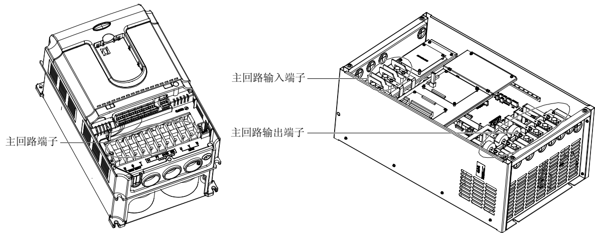
图4-2 主回路端子位置示意图
