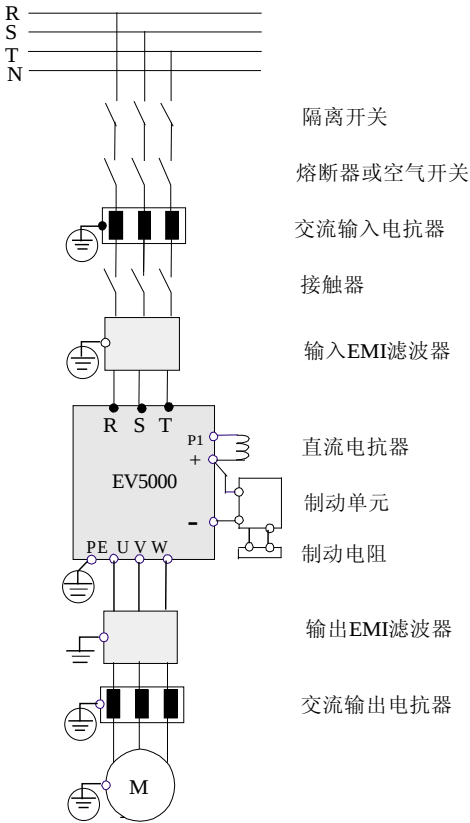
图4-3 变频器与选配件的连接
