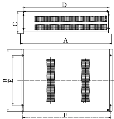
图2-10 制动电阻的安装尺寸示意图
