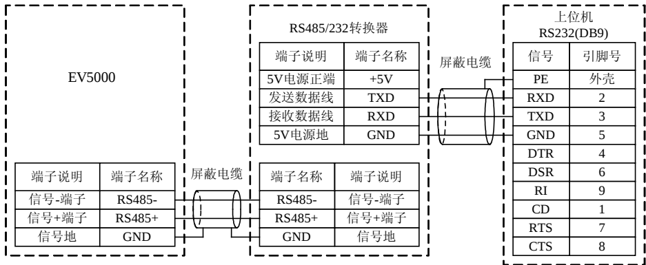
图4-18 RS485- (RS485/232) -RS232 通讯配线
