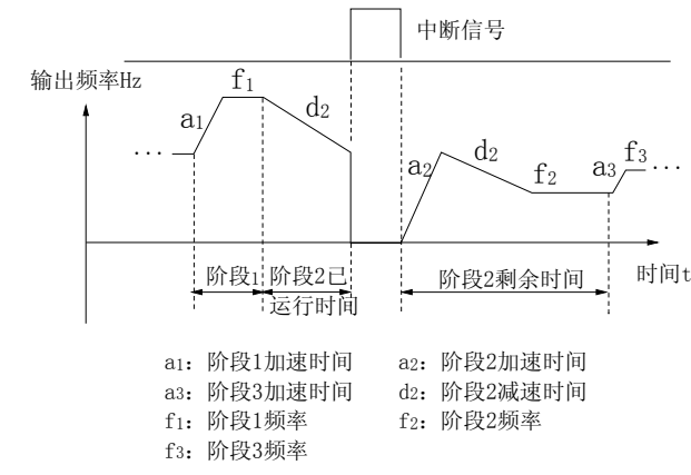
图6-42 PLC 起动方式 2
