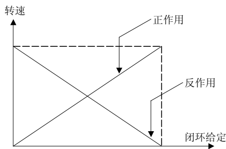
图6-47 闭环调节特性示意图
