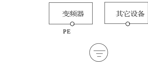
图4-41 接地示意图 2
