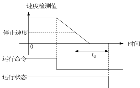
图6-30 停止速度检测时序
