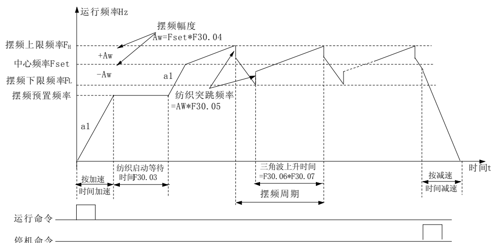
图6-95 摆频示意图
