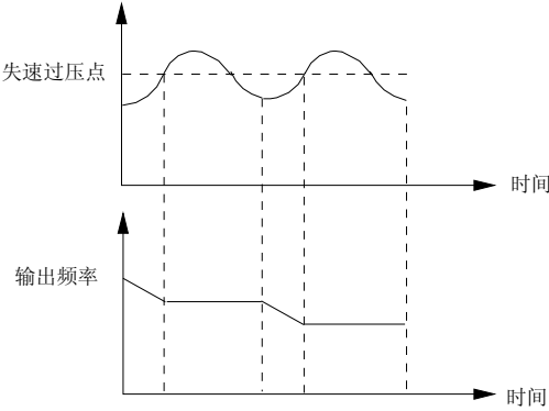
图6-88 过压失速功能
