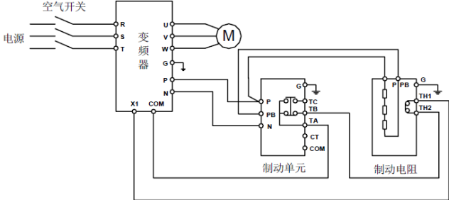
图2-11 变频器与制动组件连线图
