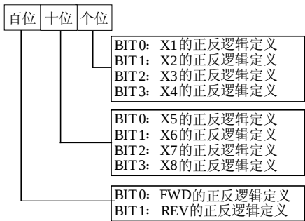
图6-61 端子正反逻辑设定
