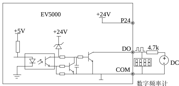
图4-30 输出端子 DO 连接方式 2
