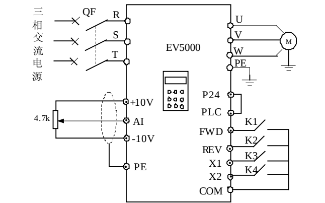
图6-24 两地控制硬件接线图
