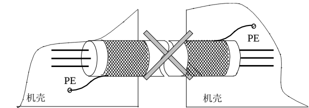
图4-39 错误的屏蔽接地方法
