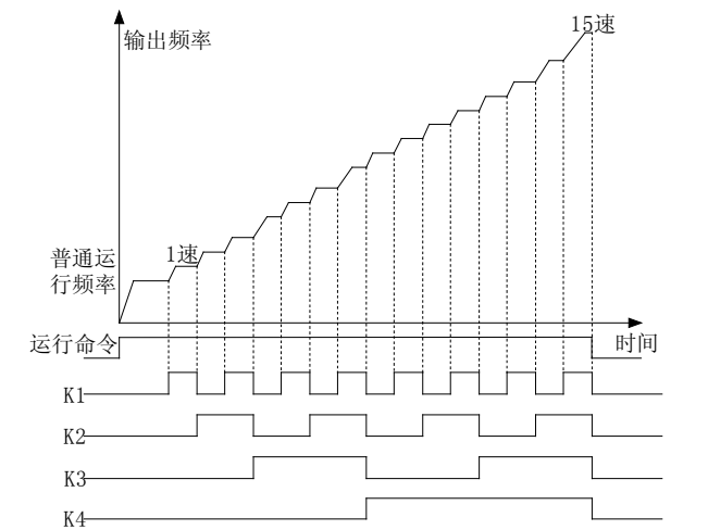
图6-52 多段速运行示意图
