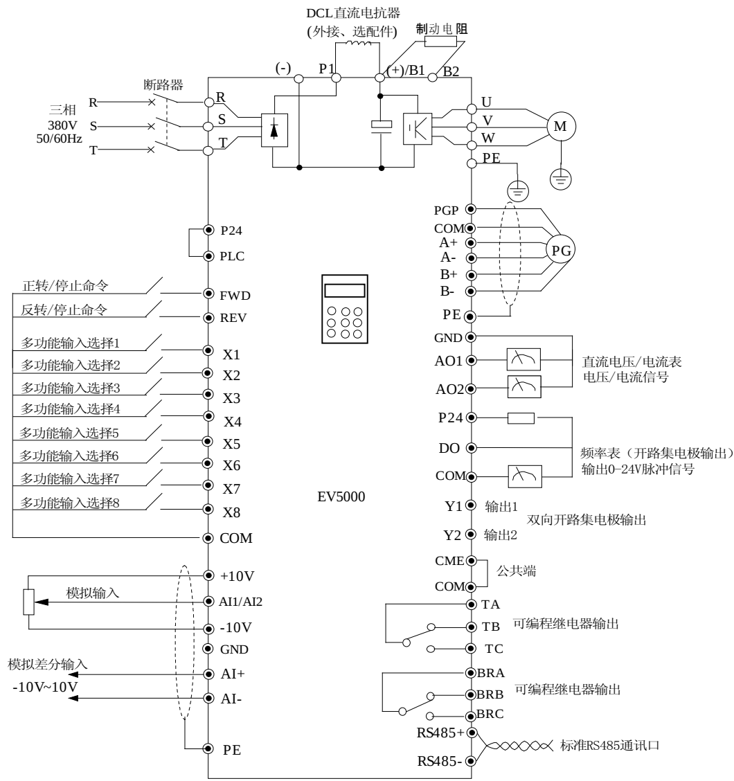
图4-4 基本配线图
