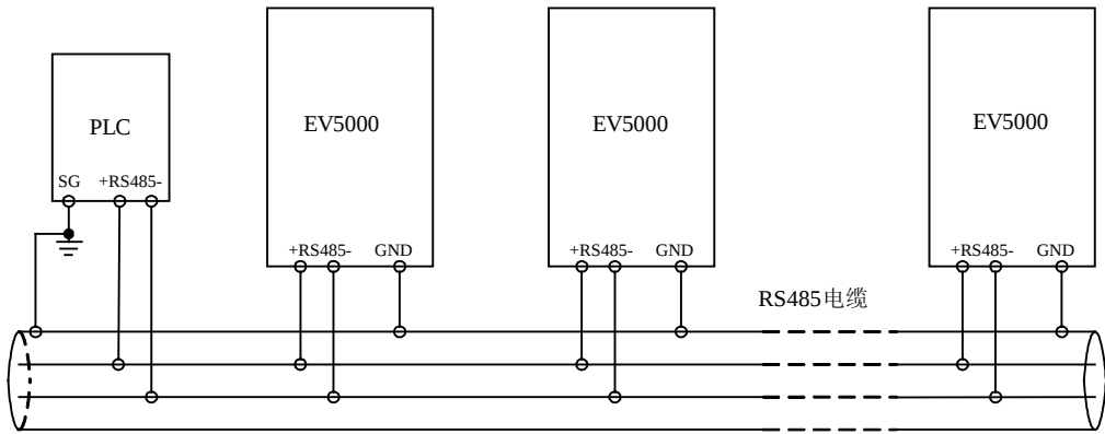
图4-20 PLC 与变频器多机通讯时推荐的接线图（变频器、电机全部良好接地）
