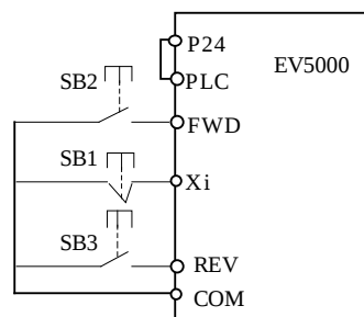
图6-56 三线式运转模式 1
