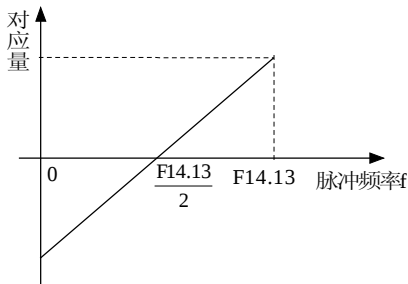
图6-60 中心点模式 2
