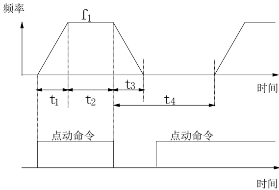
图6-21 点动运行参数说明
