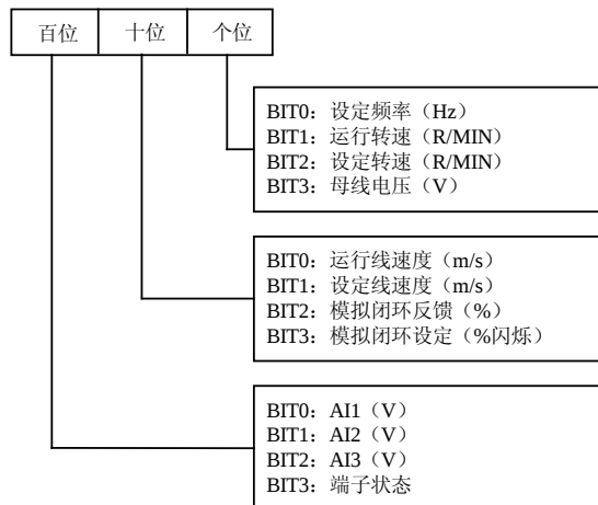
图6-84 LED 停机显示参数选择设定
