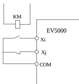
图6-53 外部设备故障常开/常闭输入示意图
