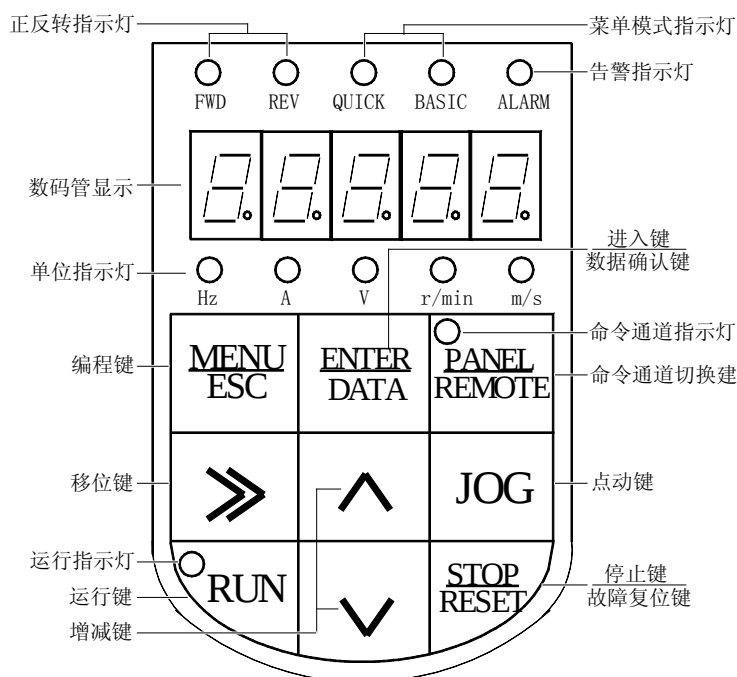
图5-1 LED 操作面板示意图
