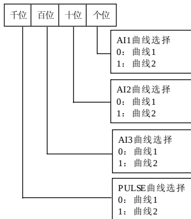
图6-14 频率给定曲线选择
