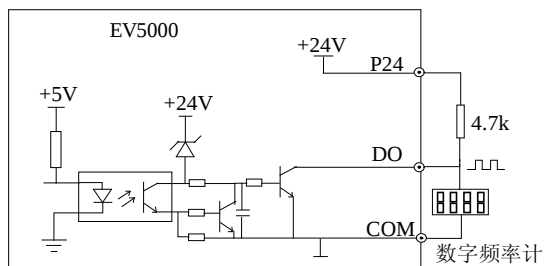
图4-29 输出端子 DO 连接方式 1
