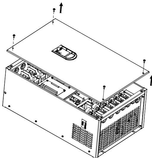
图3-7 盖板的拆卸和安装示意图
