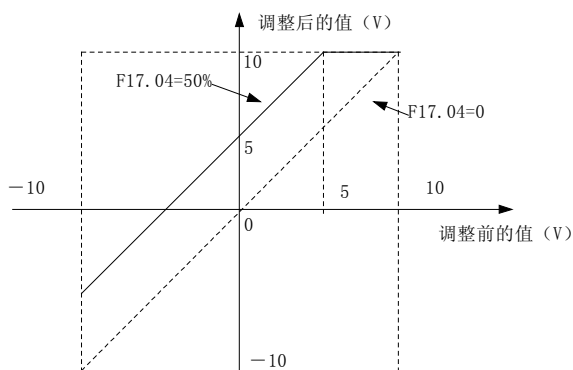
图6-80 模拟输出与零偏关系曲线
