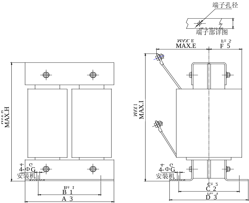
图2-5 直流电抗器的外形图
