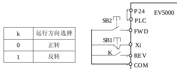
图6-57 三线式运转模式 2
