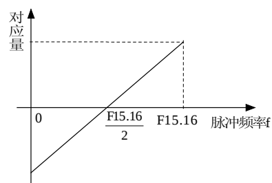
图6-68 中心点模式 2
