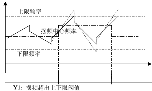
图6-62 摆频幅度限制
