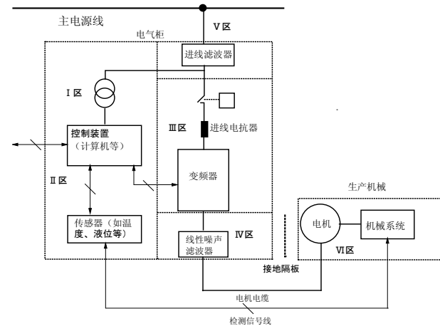
图4-46 变频器 EMC 安装推荐区域划分示意图
