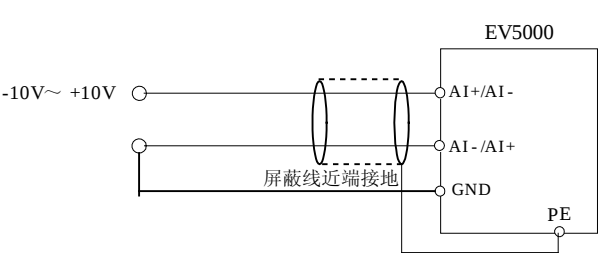
图4-15 AI+, AI-端子单端电压输入配线图
