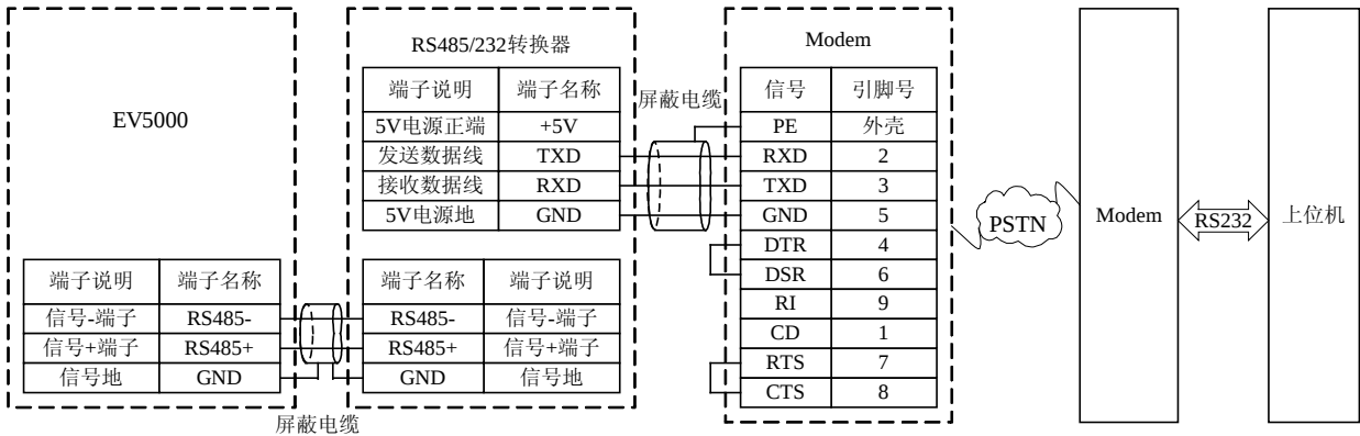
图4-19 RS485- (RS485/232) - (Modem-公网-Modem) -RS232 通讯配线
