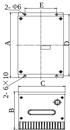
图2-9 制动单元的安装尺寸示意图
