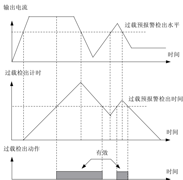
图6-90 过载预警检出功能示意图
