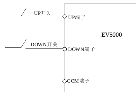
图6-7 数字设定 2 方式时，接线示意图
