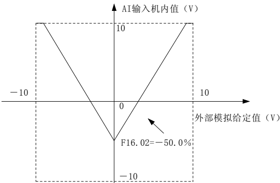
图6-77 以零偏为中心取绝对值校正模式
