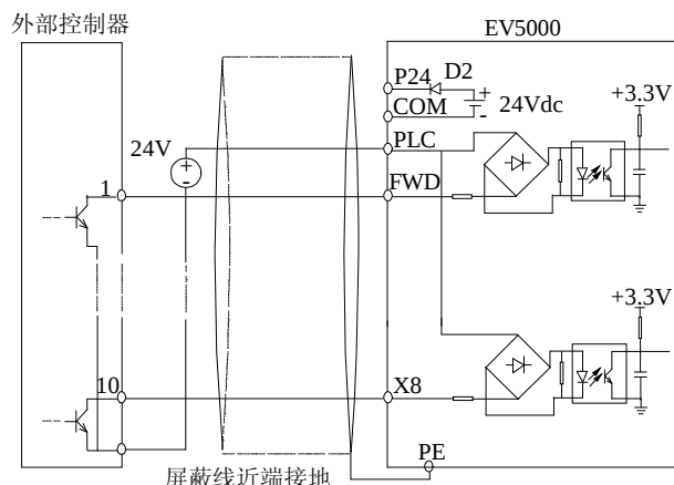
图4-25 使用外部电源的源极连接方式
