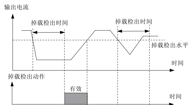
图6-91 掉载保护检出功能示意图
