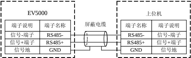
图4-17 RS485-RS485 通讯配线
