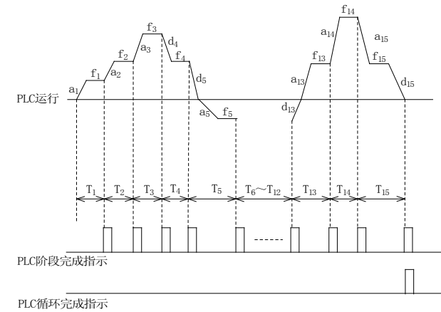
图6-36 简易 PLC 运行图
