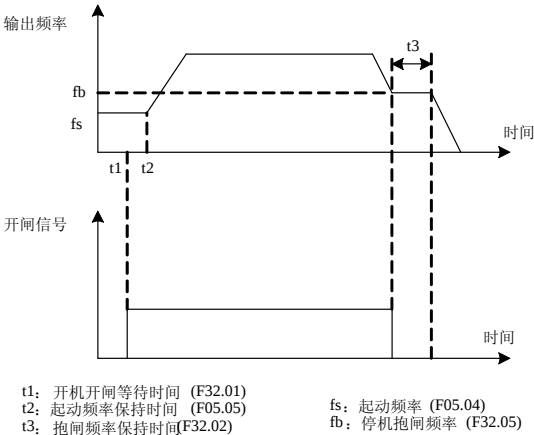
图6-97 开闸抱闸示意图
