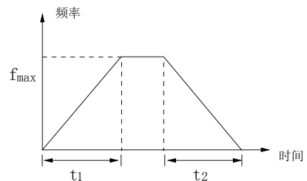
图6-17 直线加减速
