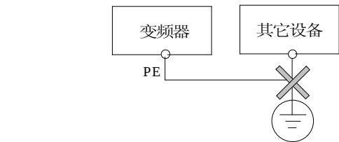
图4-42 接地示意图 3
