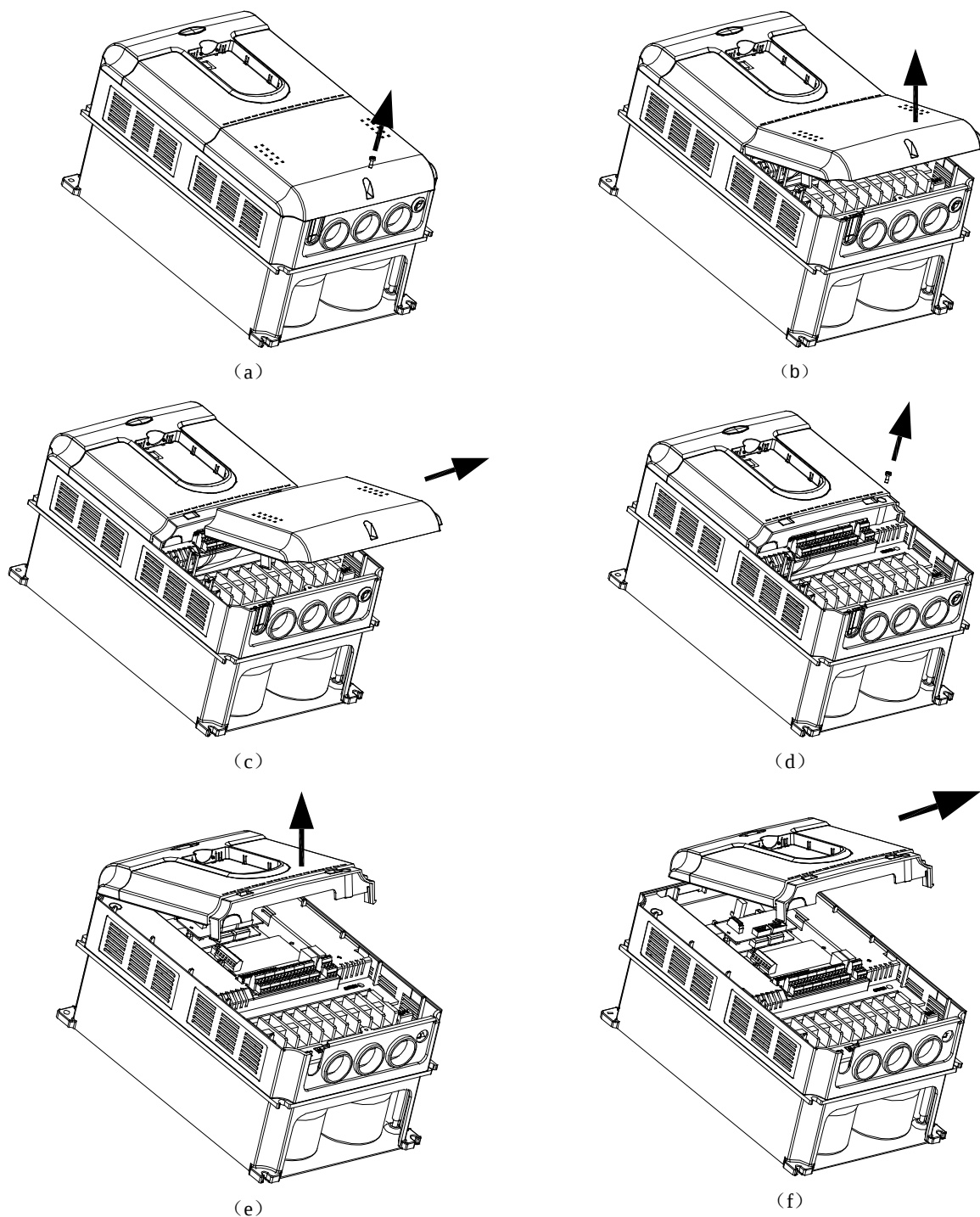
图3-6 塑胶盖板的拆卸和安装示意图
