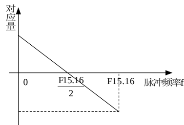
图6-67 中心点模式 1
