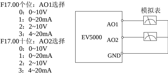
图4-16 模拟输出端子配线
