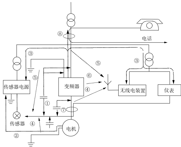
图4-36 噪声传播路径示意图
