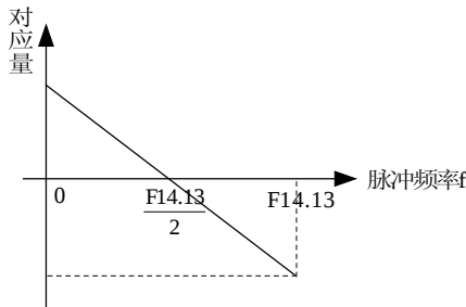
图6-59 中心点模式 1
