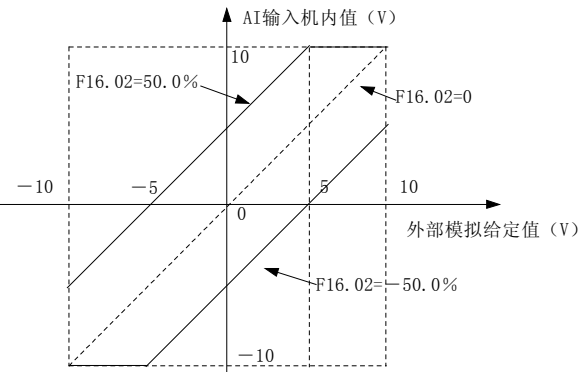
图6-73 模拟输入与零偏关系曲线
