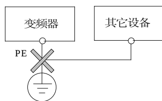
图4-43 接地示意图 4
