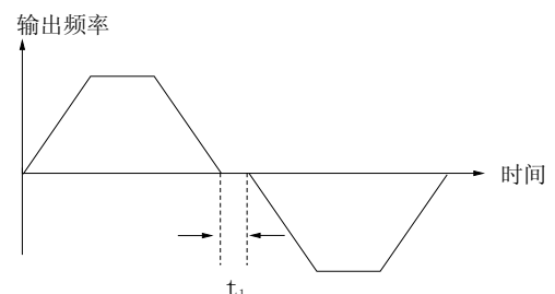
图6-29 正反转死区时间
