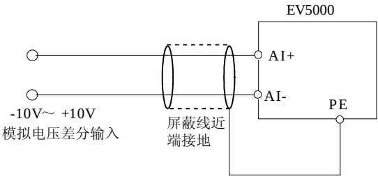
图4-14 AI+, AI-端子差分电压输入配线图
