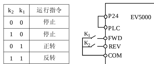
图6-55 两线式运转模式 2
