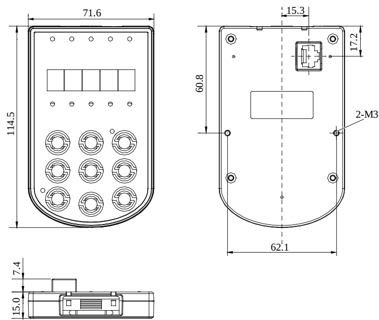
图2-6 操作面板尺寸
