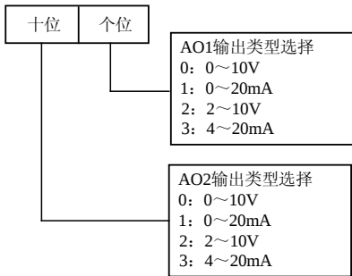
图6-78 模拟输出类型选择
