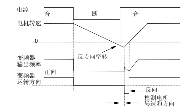
图6-25 转速跟踪再启动示意图
