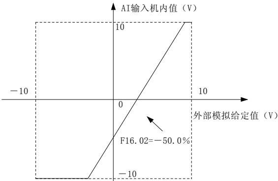
图6-74 以零偏为中心校正模式
