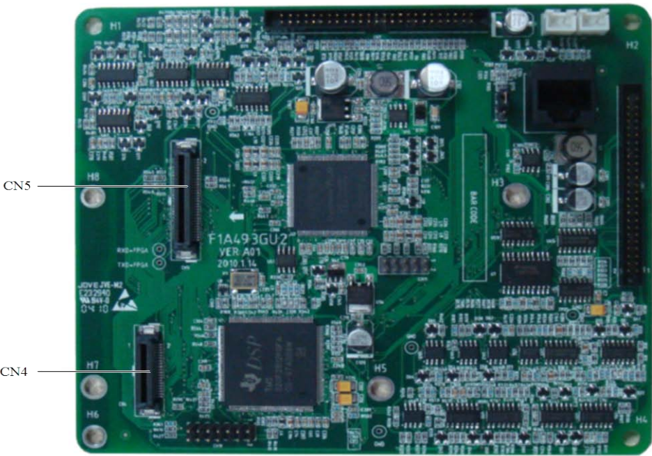
图4-34 选配件端子座位置示意图
