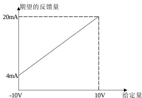
图6-46 给定量和期望反馈量
