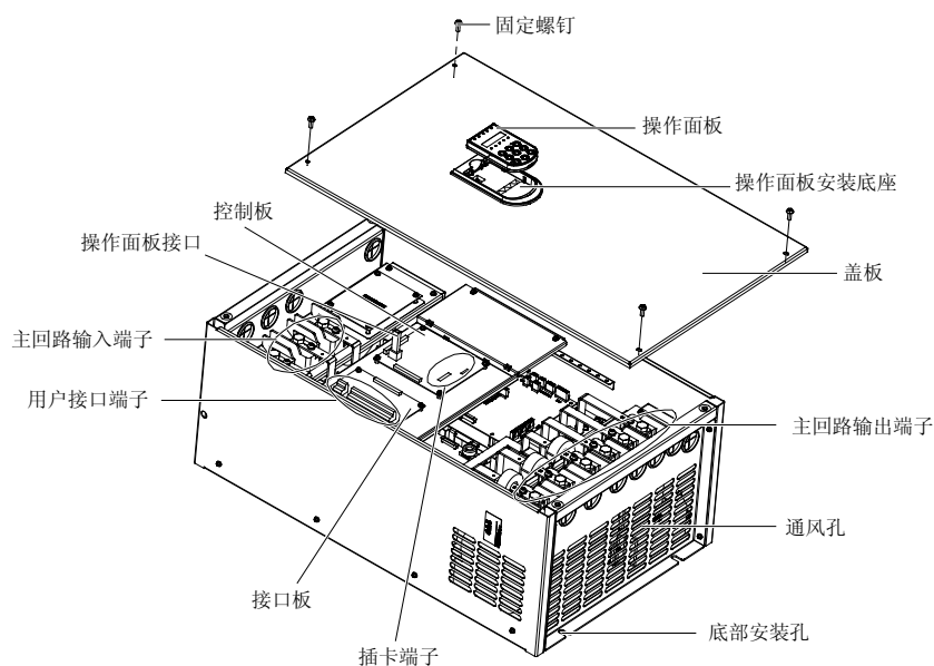
图2-2 30kW 及其功率等级以上变频器结构图
