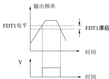
图6-65 频率水平检测示意图
