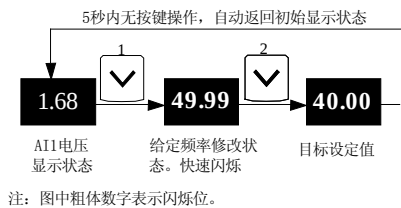
图5-6 设定设定频率操作示例
