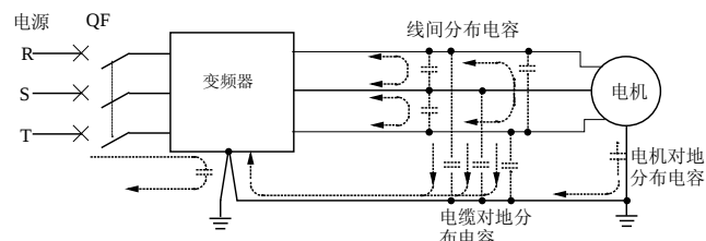
图4-45 漏电流路径
