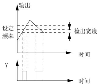
图6-64 频率到达信号输出示意图
