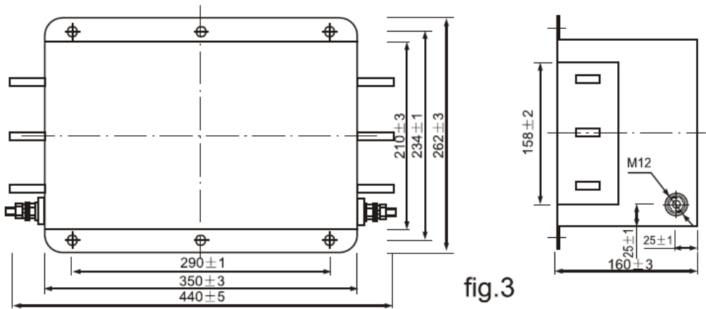
图7 300~600A EMI 滤波器外形图
