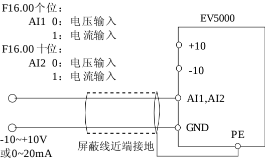
图4-13 AI1, AI2 端子配线图
