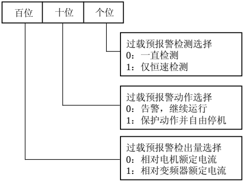
图6-89 过载预警检出选择
