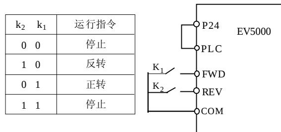
图6-54 两线式运转模式 1
