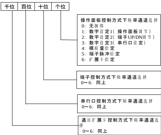
图6-22 运行命令通道捆绑频率给定通道
