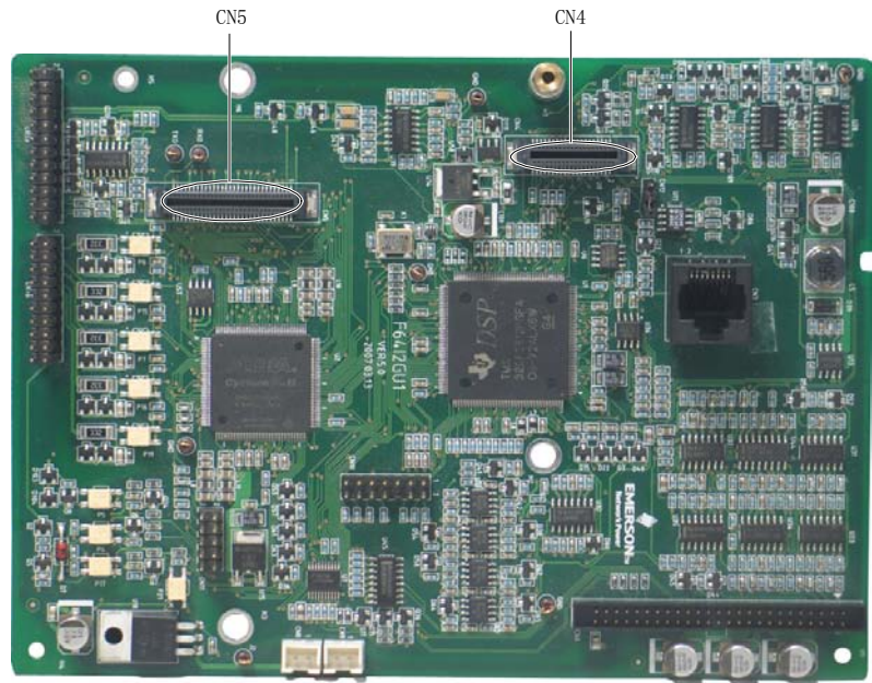
图4-33 选配件端子座位置示意图
