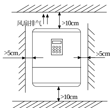
图3-1 安装的间隔距离（45kW 及以下）
