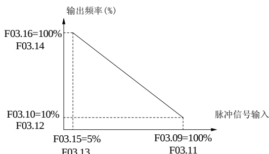
图6-16 脉冲信号输入实例参数设置 2
