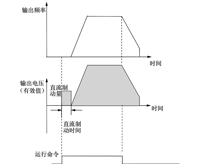
图6-27 起动方式 1 说明
