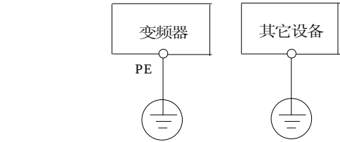
图4-40 接地示意图 1
