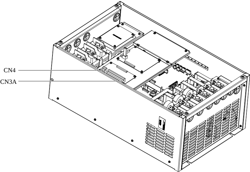
图4-8 控制回路端子在变频器上的位置示意图
