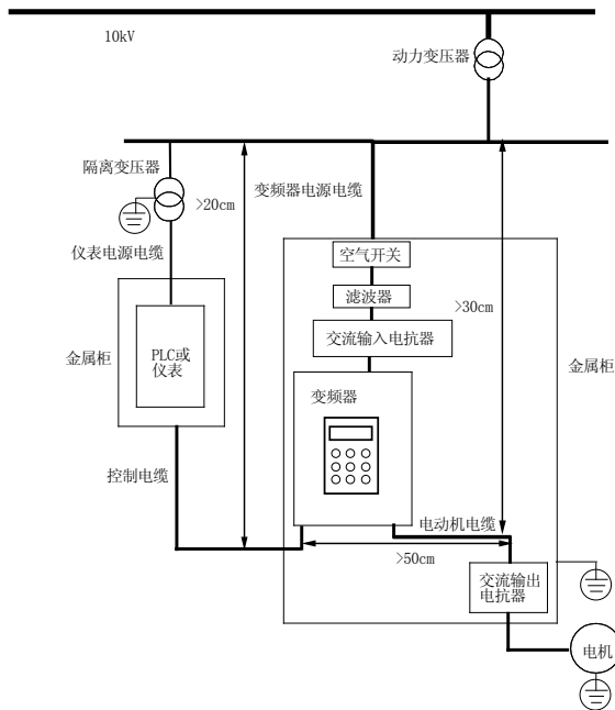
图4-47 变频器的安装示意图
