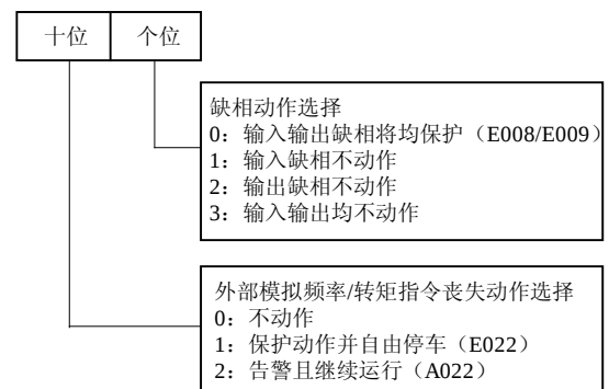
图6-86 保护动作选择 2 设定
