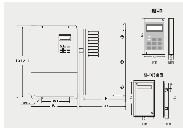
机箱规格表
