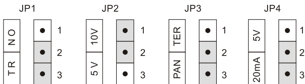
终端电阻选择跳线
