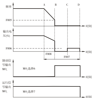
制动过程中频率及输出电压和时间的关系
