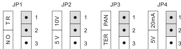
终端电阻选择跳线
