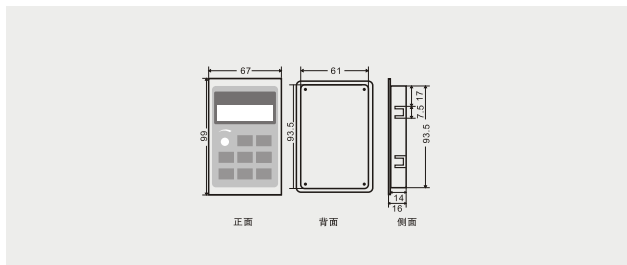
机箱规格表
