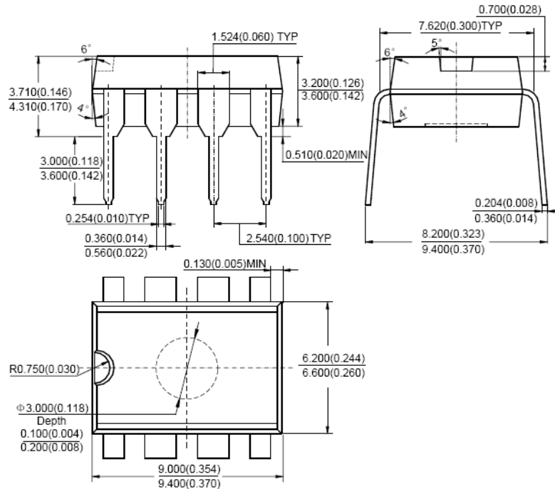
DIP-8
