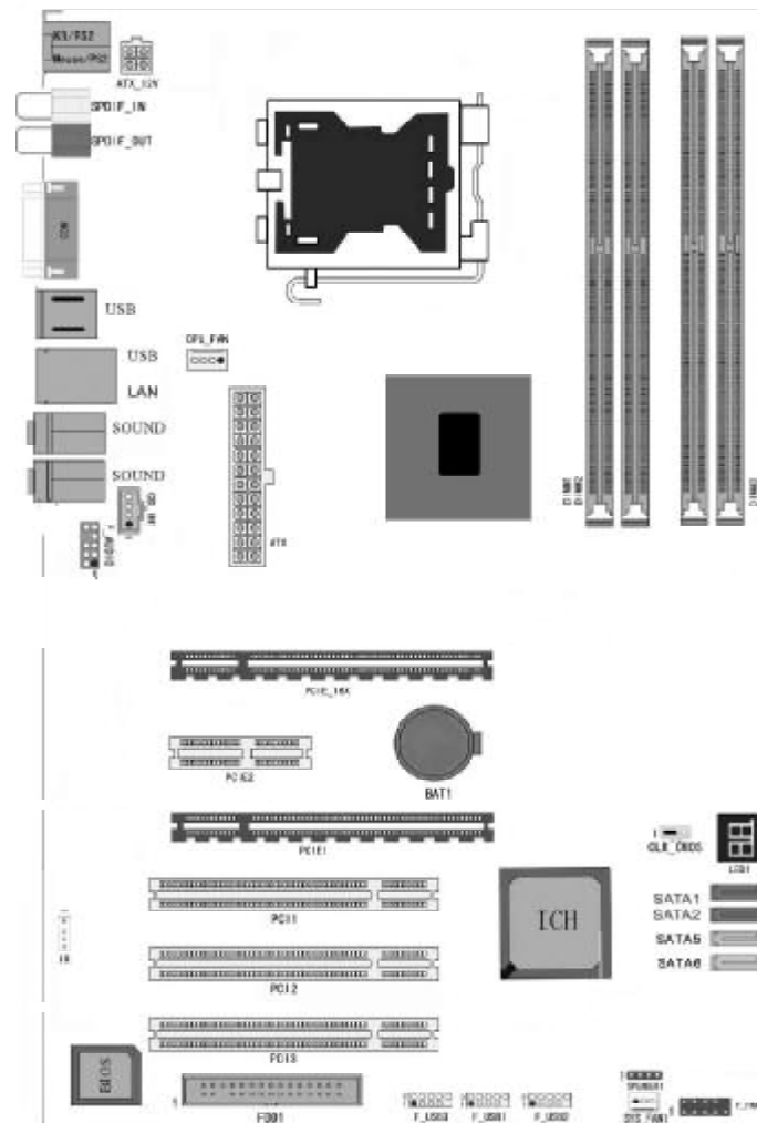
C.P965-MVP Ver2.0 主机板布局图
