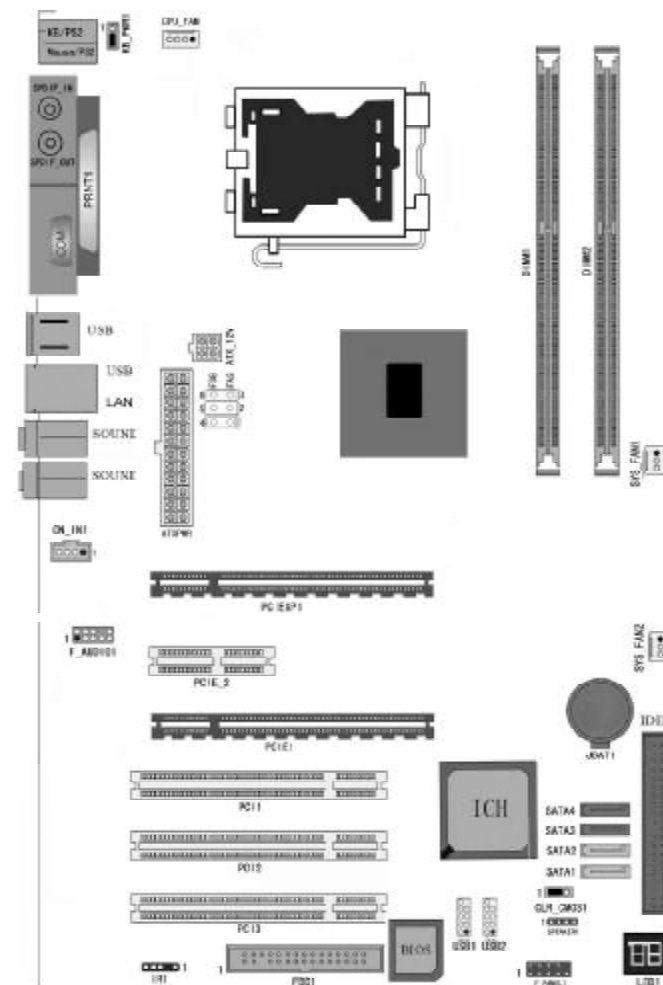
C.945P - MVP Ver2.1 主机板布局图
