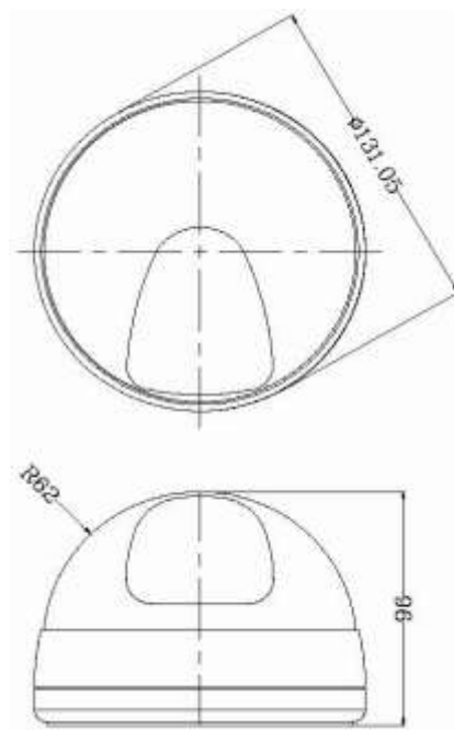
2.1-1-2结构尺寸图
