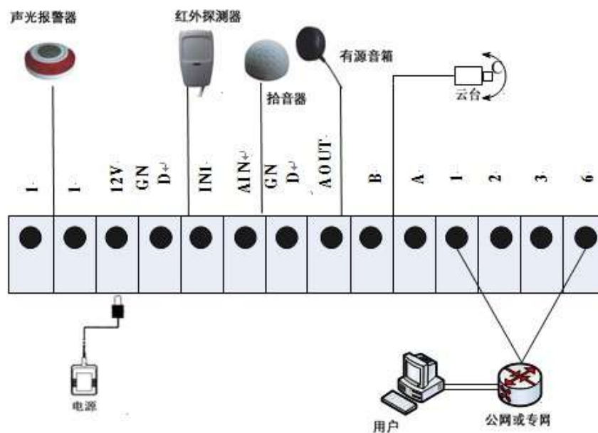
图 3.1-3 硬件连接图
