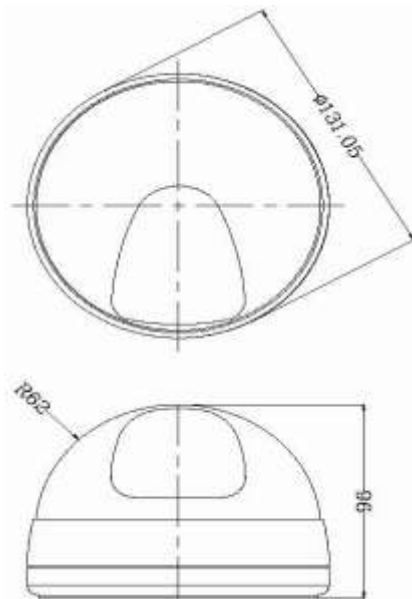
图 2.1-1 外观图
