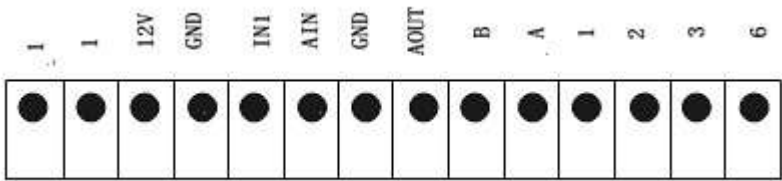
图 2.1-3 用户接口图
