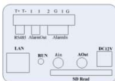
图 2.1-3 用户接口图
