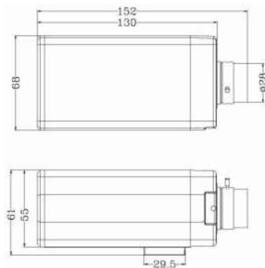
2.1-1-2结构尺寸图
