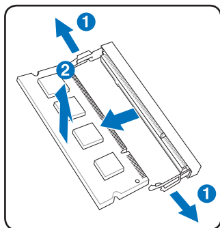
移除内存条
