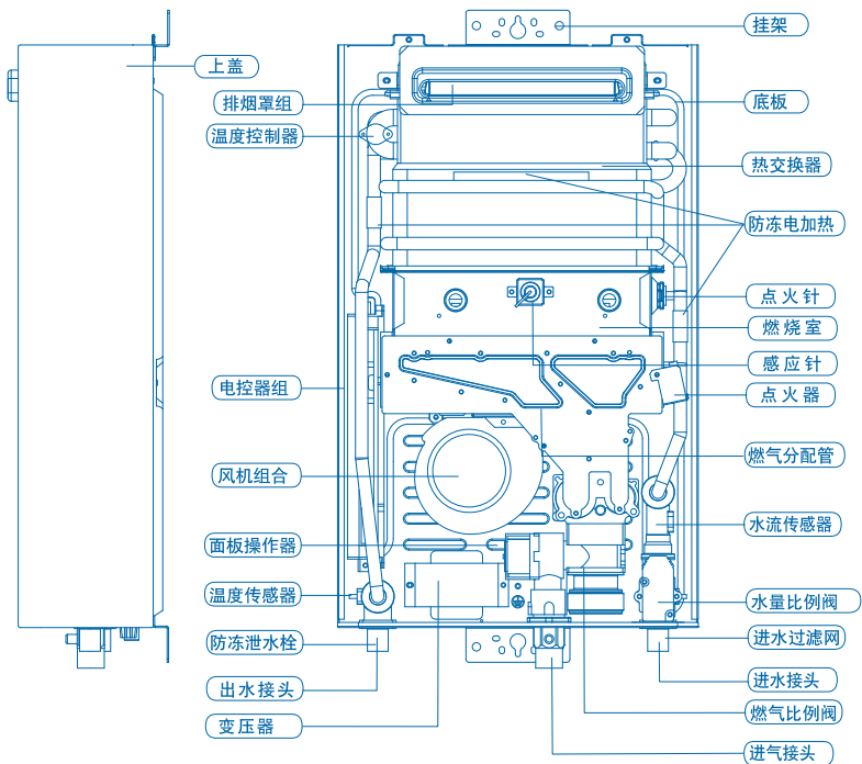
b. JSW32-Hi7/JSW32-Hi7S机型:
