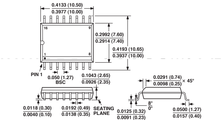
16-Lead SOIC (S Suffix)
