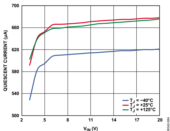
图22. 静态电流与 V_{IN} 的关系
