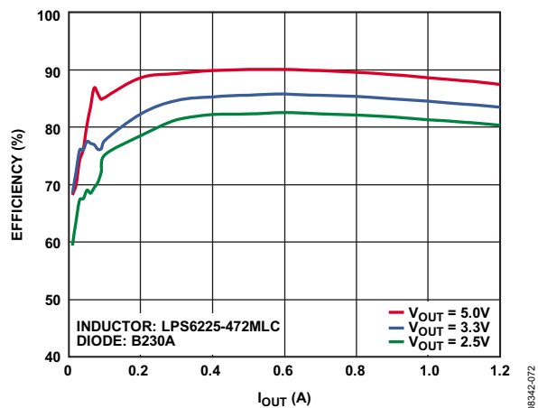
图6. 功效曲线, V_{IN} = 12\text{ V} , f_{SW} = 1.4\text{ MHz}
