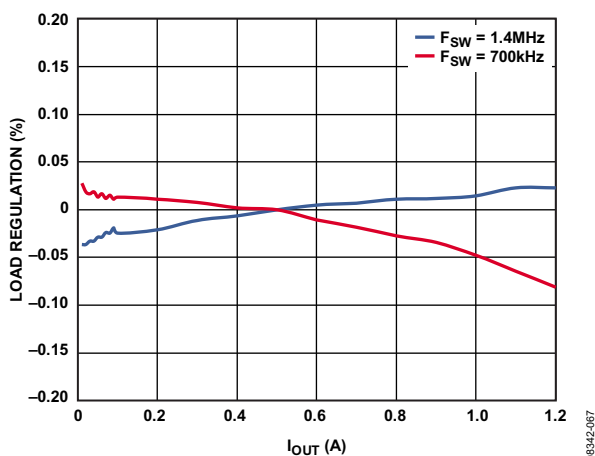
图12. 负载调整率, V_{OUT} = 3.3V , V_{IN} = 12V
