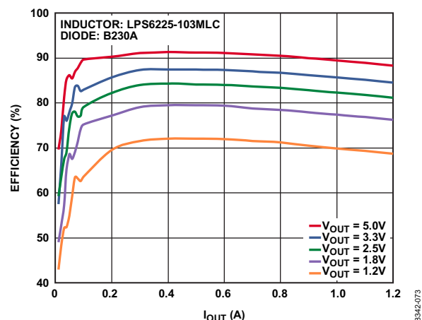
图7. 功效曲线, V_{IN} = 12\text{ V} , f_{SW} = 700\text{ kHz}
