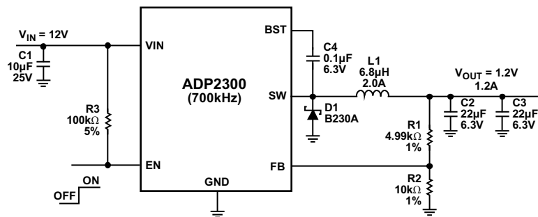
图51. ADP2300—700kHz典型应用, V_{IN}=12V , V_{OUT}=1.2V/1.2A , 带外部使能
