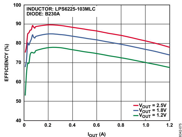
图9. 功效曲线, V_{IN} = 5.0\text{ V} , f_{SW} = 700\text{ kHz}
