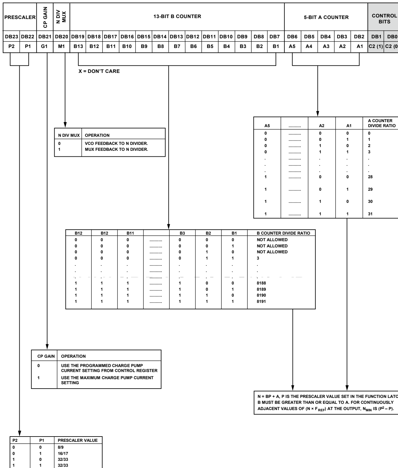
Figure 25. LO Latch
