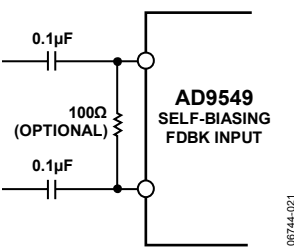
Figure 21. FDBK Input
