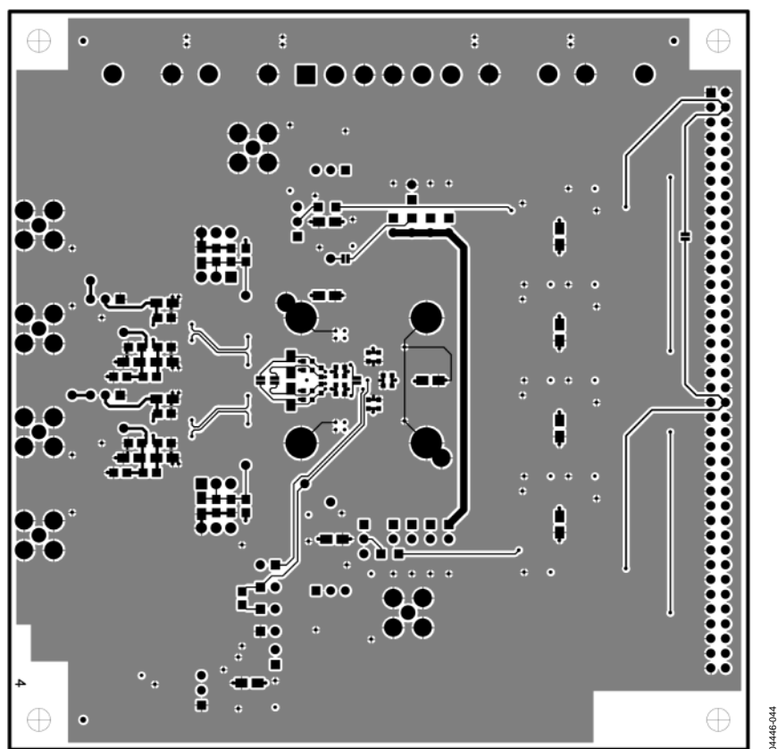
Figure 44. Bottom Layer
